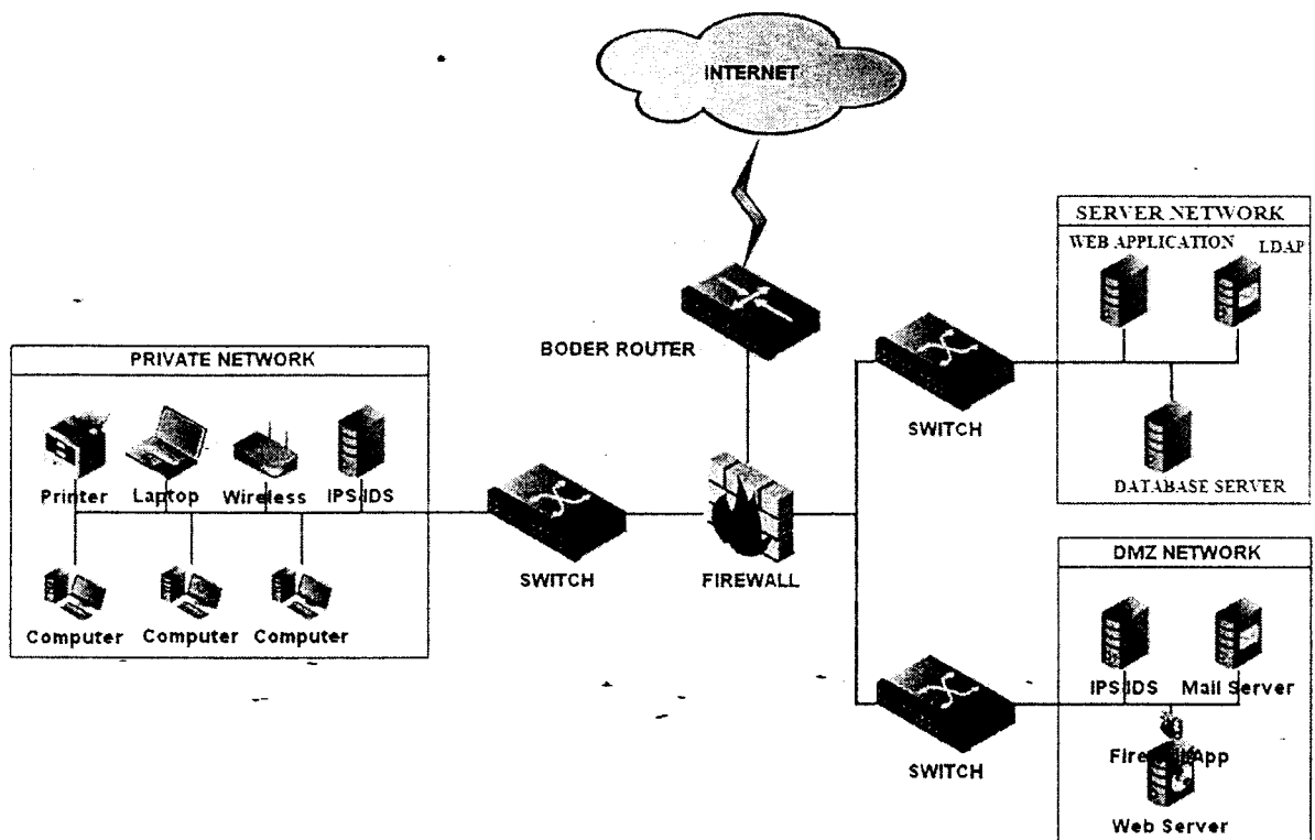
Hình 3. Mô hình mạng tổng quan
