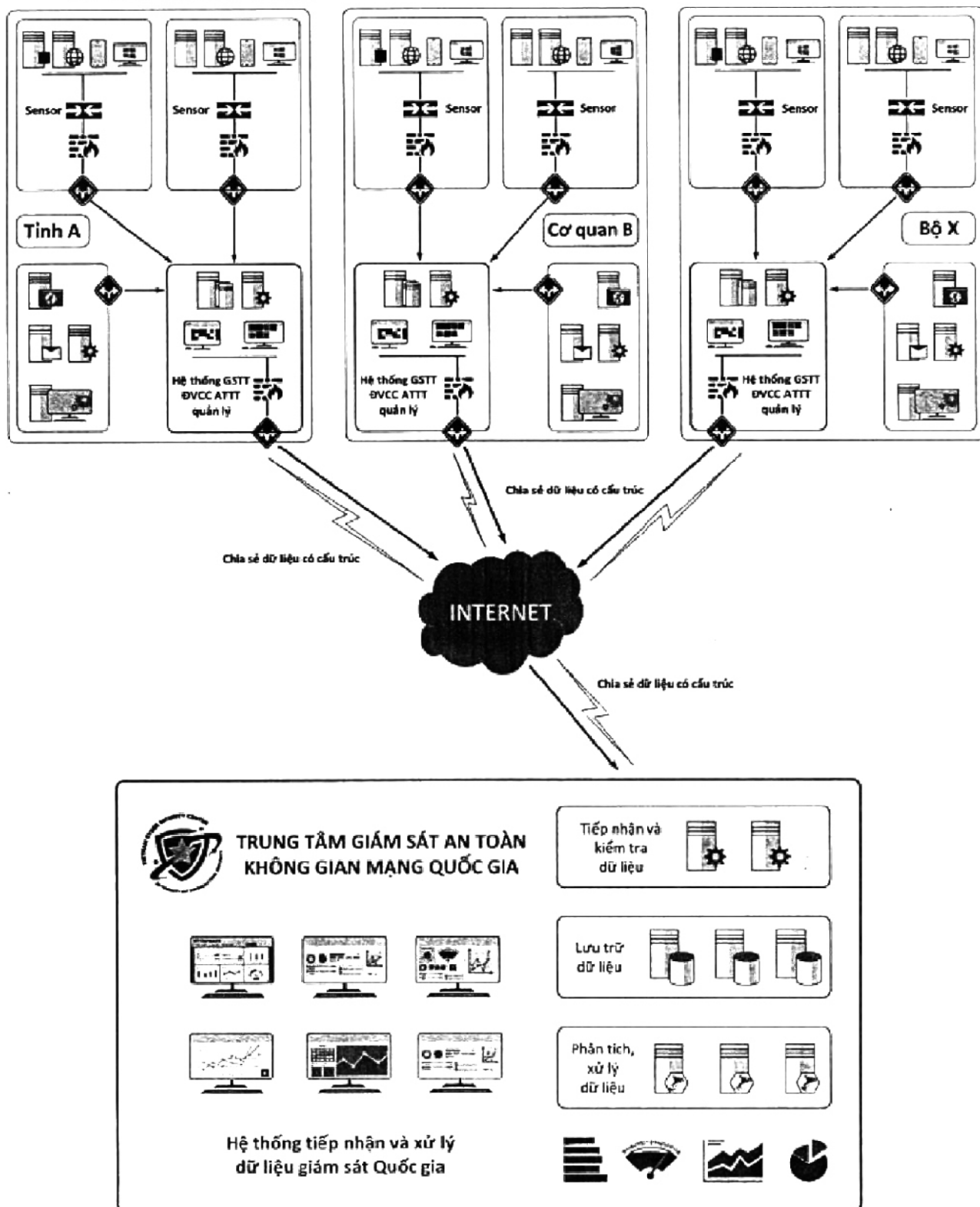
Hình 4. Mô hình kết nối hệ thống
