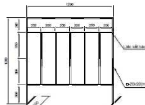
RÀO CHẮN DI ĐỘNG BẢNG KHUNG THÉP HÌNH MẪU B-3
