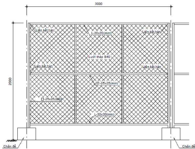
CHI TIẾT RÀO CHẮN
