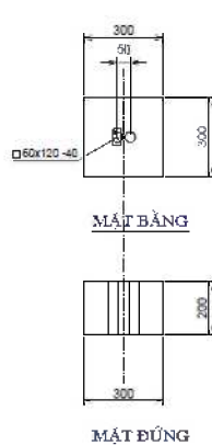
CHI TIẾT CHÂN ĐẾ RÀO CHẮN MẪU C-1
