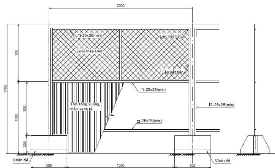
CHI TIẾT THÂN RÀO CHẮN (MẪU K-4)
