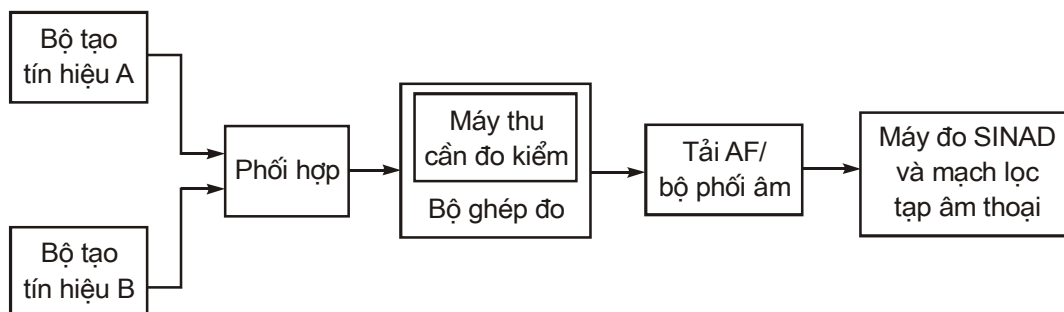
Hình 14 - Sơ đồ đo độ triệt nhiễu cùng kênh
