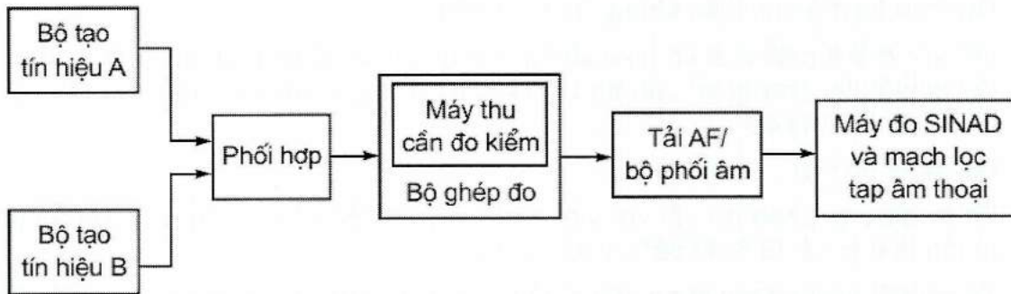
Hình 14 - Sơ đồ đo độ chọn lọc kênh lân cận
