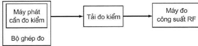
Hình 5 - Sơ đồ đo trong điều kiện đo kiểm tới hạn
