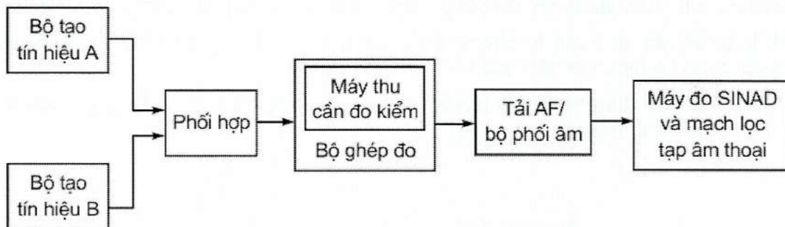
Hình 13 - Sơ đồ đo triệt nhiễu đồng kênh
