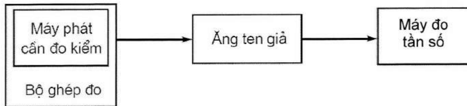
Hình 2 - Sơ đồ đo sai số tần số
