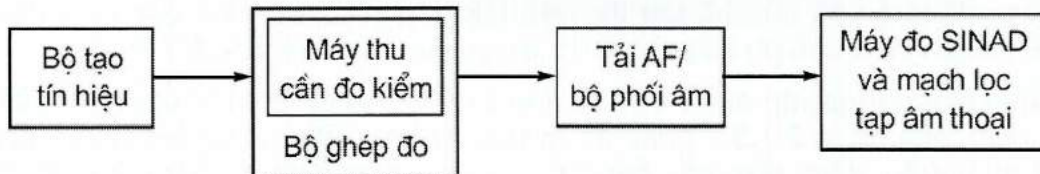
Hình 12 - Sơ đồ đo trong điều kiện đo kiểm tới hạn
