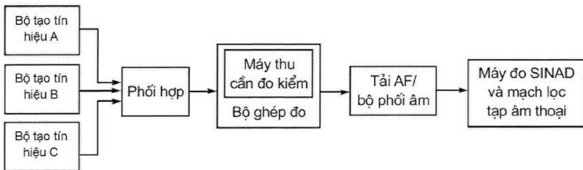
Hình 16 - Sơ đồ đo triệt đáp ứng xuyên điều chế
