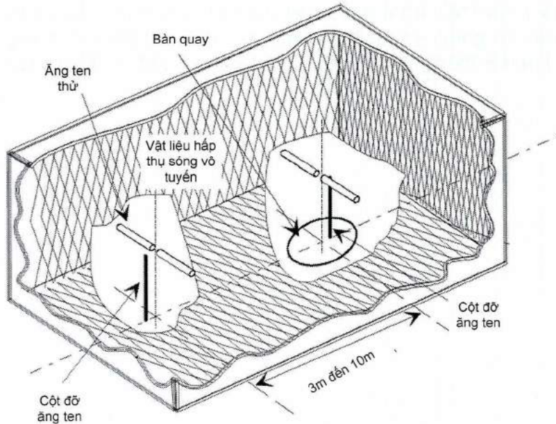
Hình A.1 - Buồng đo không phản xạ
