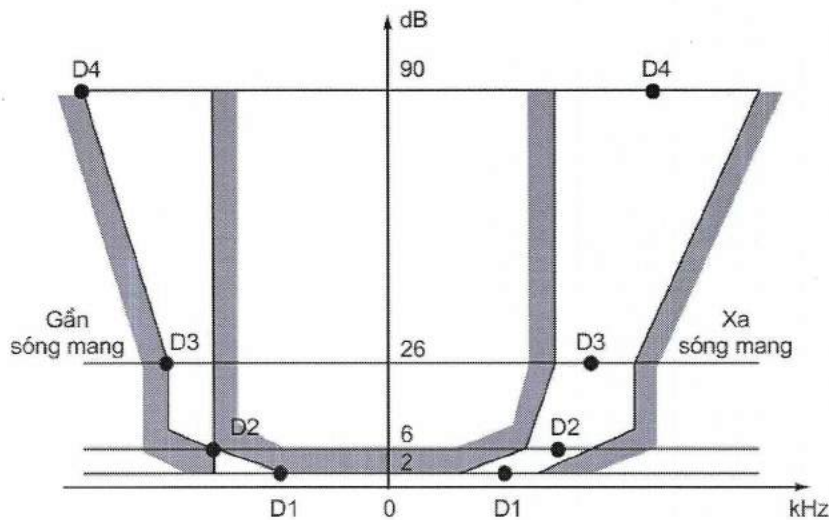
Hình B.2 - Bộ lọc IF
