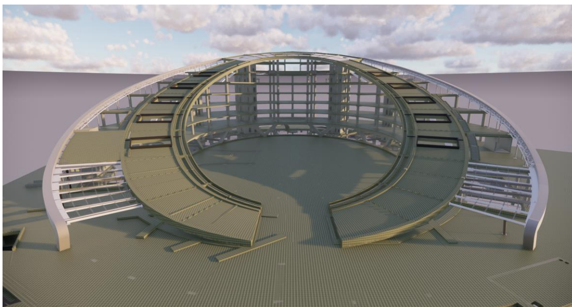
Hình 12 Mô hình kết cấu của Dự án D26 Trụ sở Viettel trong giai đoạn thiết kế cơ sở
