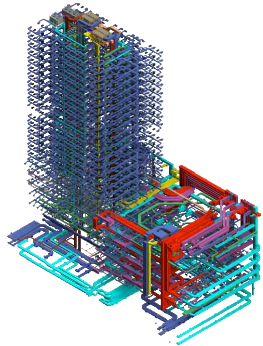
Hình 1.8 Mô hình MEP dự án Crescent Mall giai đoạn 2
