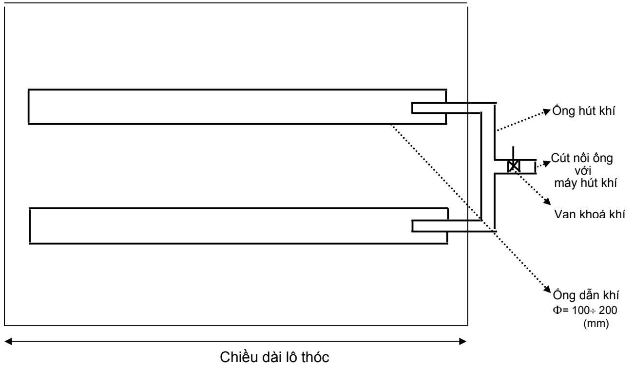
Hình 3: Mô hình hệ thống ống dẫn, hút khí kho A1
