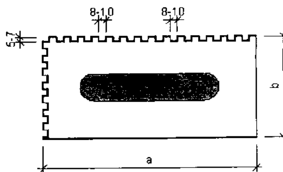
Hình C.12 - Bàn gạt vữa
