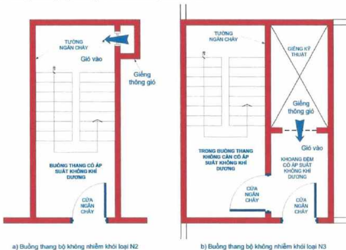
Hình I.9 - Minh họa buồng thang bộ không nhiễm khói loại N2 và N3
