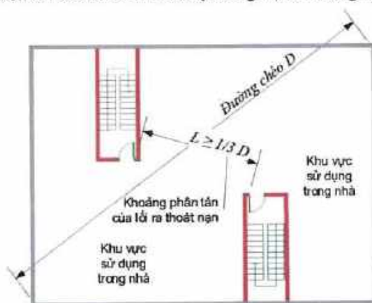
Hình I.4 - Nguyên tắc nửa đường chéo mặt bằng khi bố trí phân tán các lối ra thoát nạn
