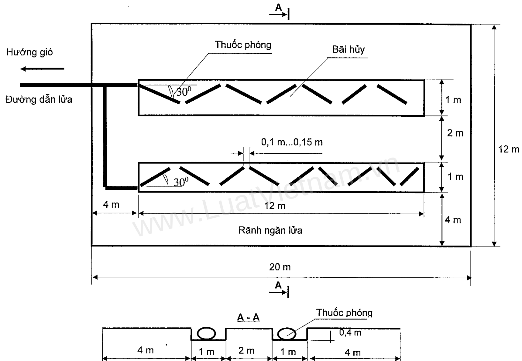
Hình B5 - Sơ đồ khu vực hủy đốt thuốc phóng đạn phản lực
