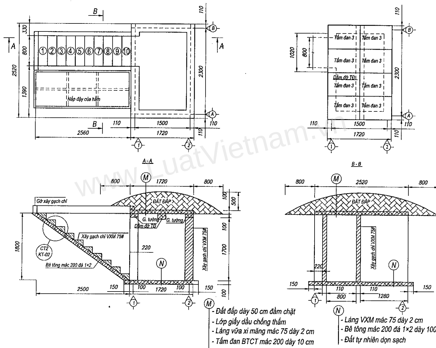
Hình A3 - Hầm để thuốc phóng chờ hủy
