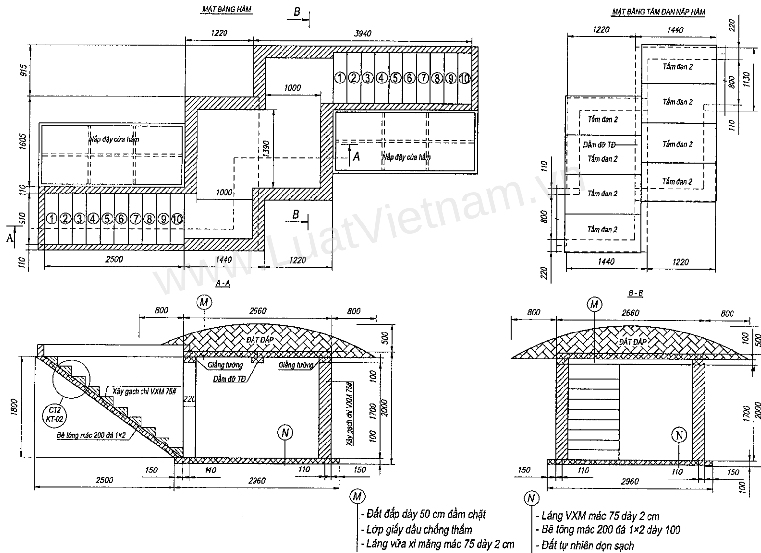
Hình A2 - Hầm chỉ huy
