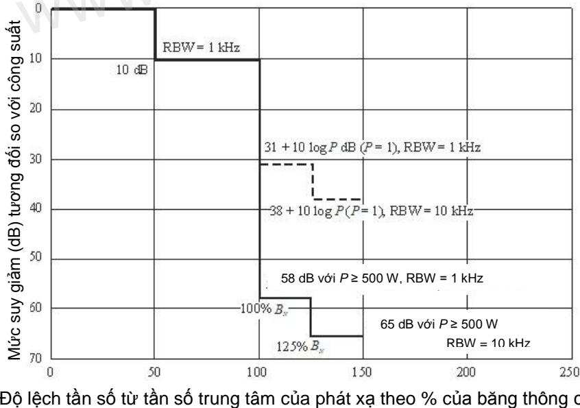
Hình D.11 - Các đòi hỏi trong dải tần trên 30 MHz trong trường hợp băng rộng của khuyến nghị ITU-R SM.1539
