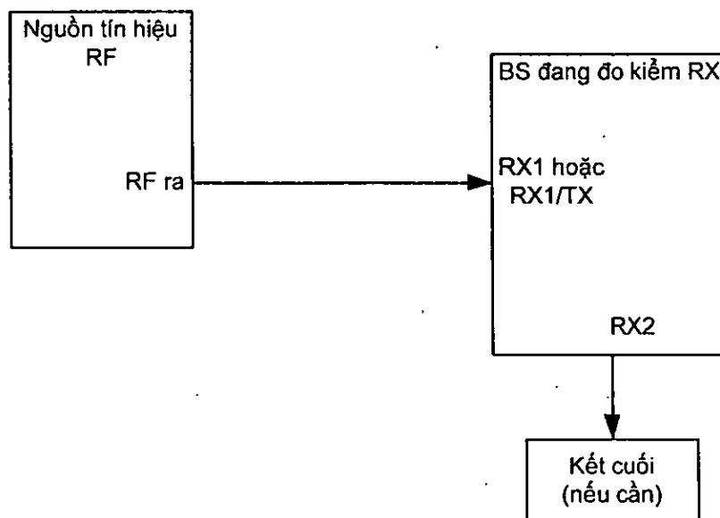
Hình C.7 – Thiết lập hệ thống đo mức chọn lọc chuẩn trạm gốc
