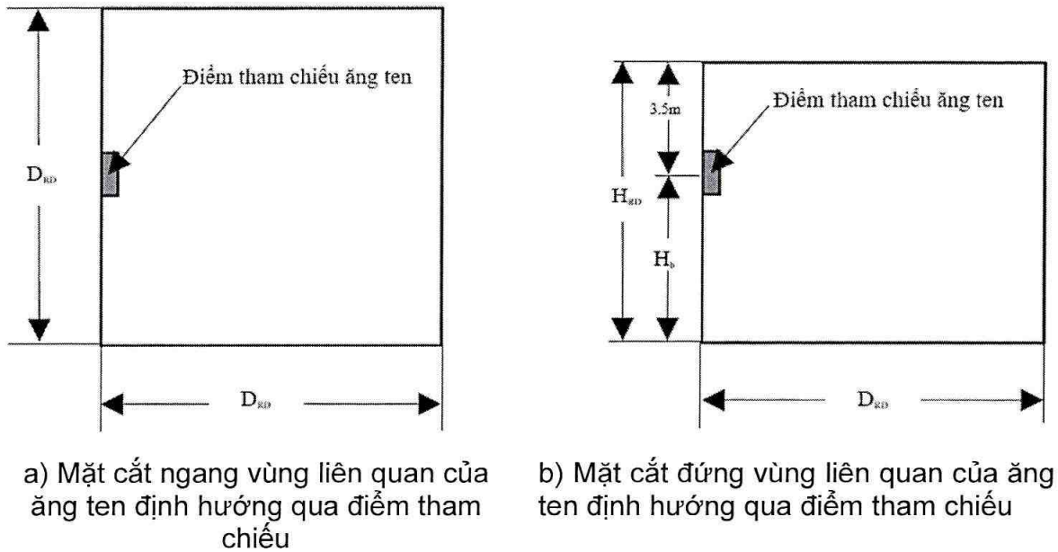
Hình B.1 - Mặt cắt vùng liên quan của ăng ten định hướng
