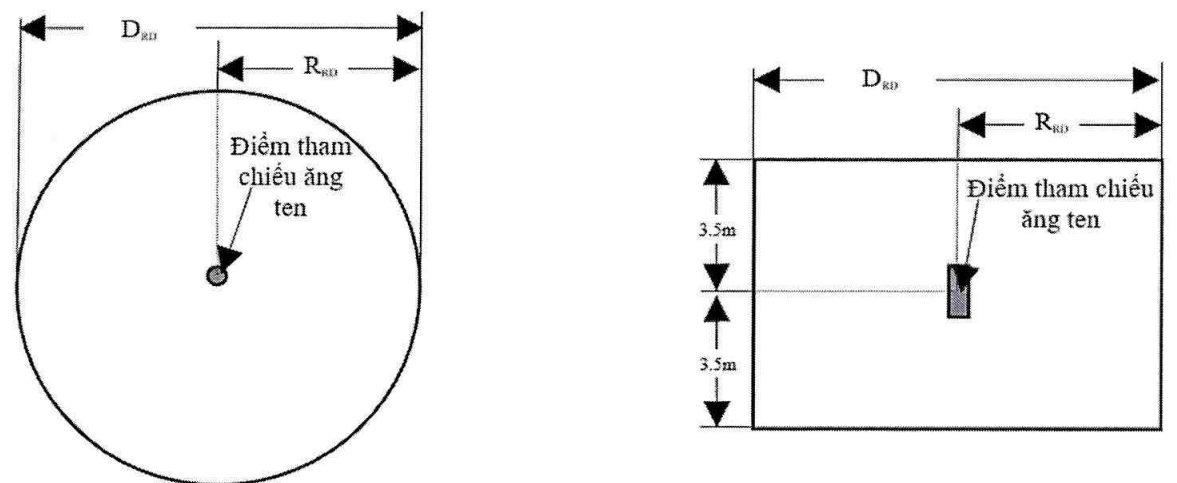
Hình B.1 - Mặt cắt vùng liên quan của ăng ten định hướng
