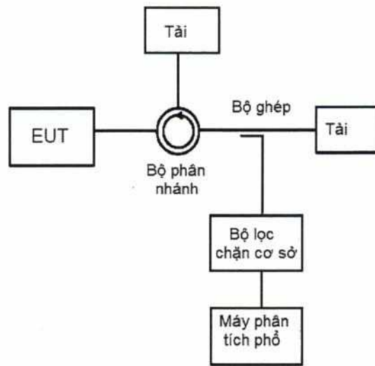
Hình 6 - Sơ đồ đo phát xạ không mong muốn truyền dẫn
