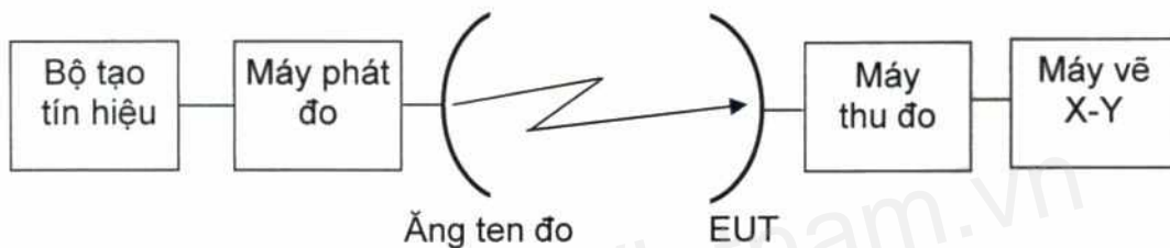
Hình 18 - Sơ đồ đo – phép đo gián tiếp thu của ăng ten
