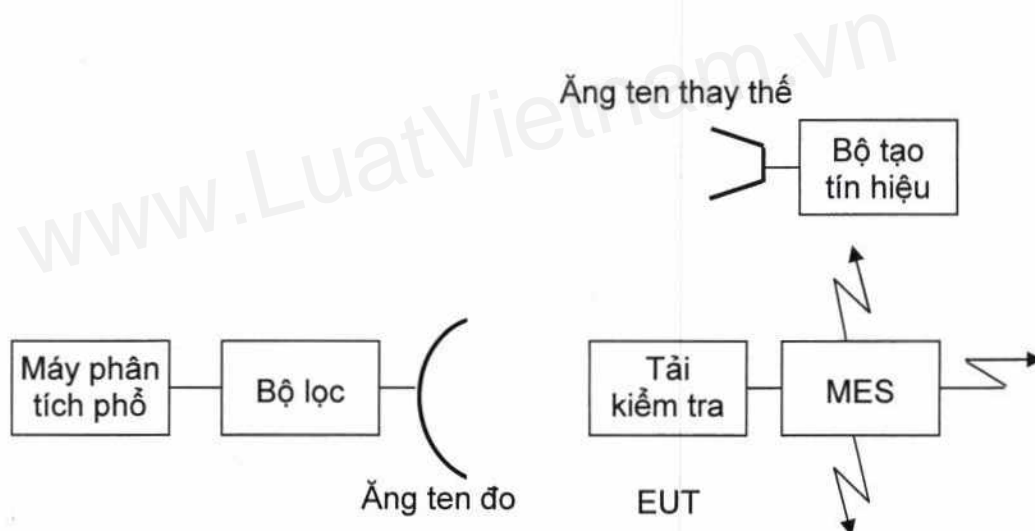
Hình 5 - Sơ đồ đo phát xạ không mong muốn của EUT khi không có ăng ten
