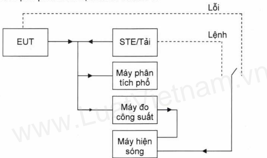
Hình 16 - Sơ đồ đo chung cho các phép đo về giám sát và điều khiển đối với những phép đo truyền dẫn
