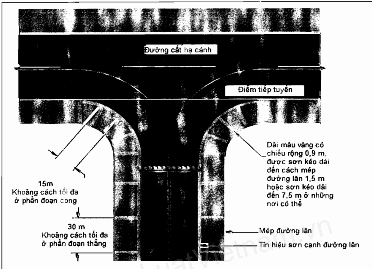
Hình 20 - Sơn tín hiệu lề đường lán (Tại nơi đường lán giao với đường CHC)
