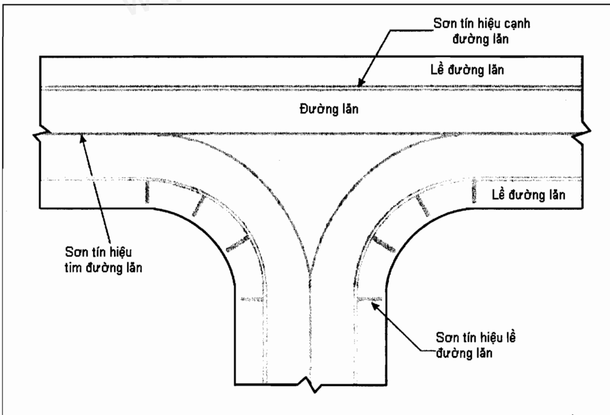
Hình 21 - Sơn tín hiệu lề đường lán (Tại nơi đường lán giao với đường lán)
