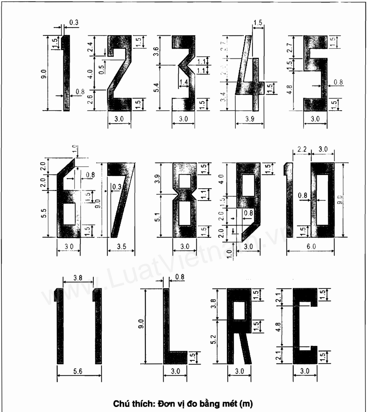
Hình 2 - Hình dạng, tỷ lệ chữ và số chỉ hướng đường cát hạ cánh
