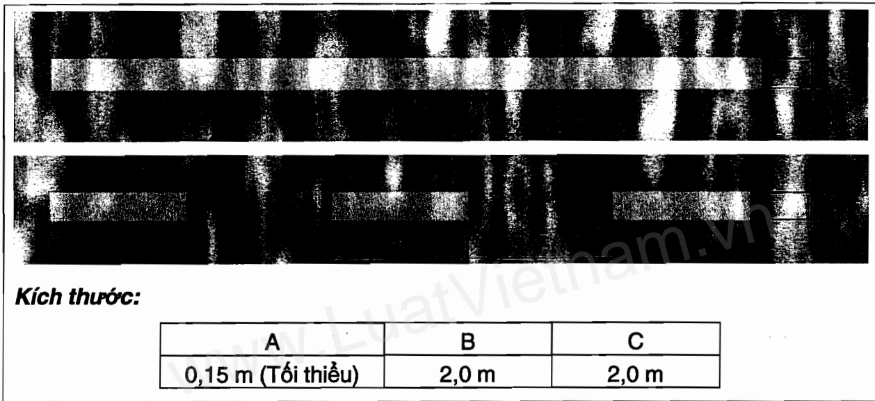
Hình 26 - Sơn tín hiệu vạch dẫn lăn
