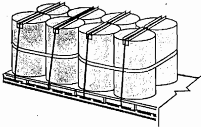
Xếp, cố định cuộn tròn đứng trên thùng xe
