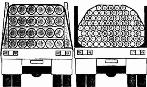
Xếp, cố định ống trụ dài trong thùng xe kín
