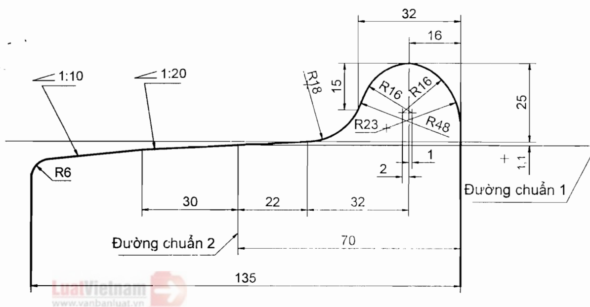
Hình 2. Biên dạng mặt lăn côn khổ đường 1.435 mm
