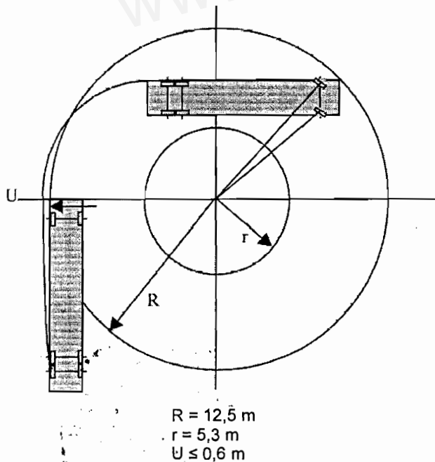
Hình 6a - Khả năng quay vòng xe thẳng liền
