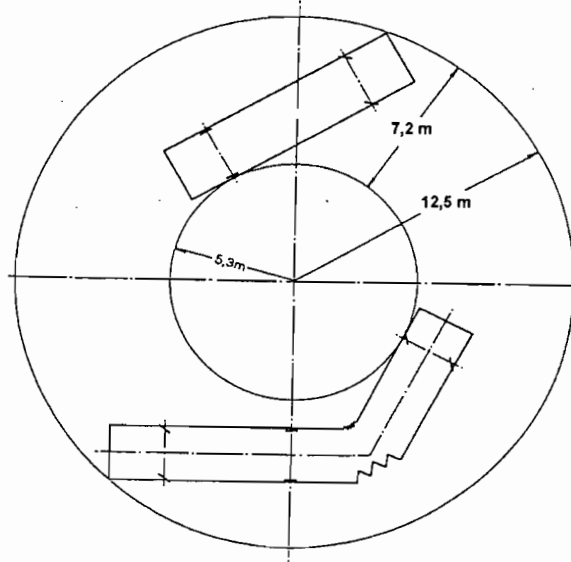
Hình 5 - Khả năng quay vòng
