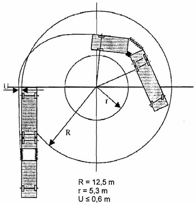
Hình 6b - Khả năng quay vòng xe nổi toa
