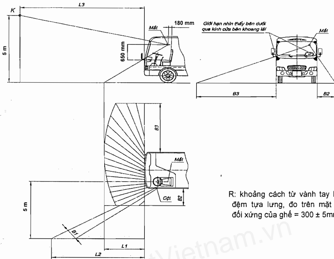
Hình 1 - Tầm nhìn của người lái
