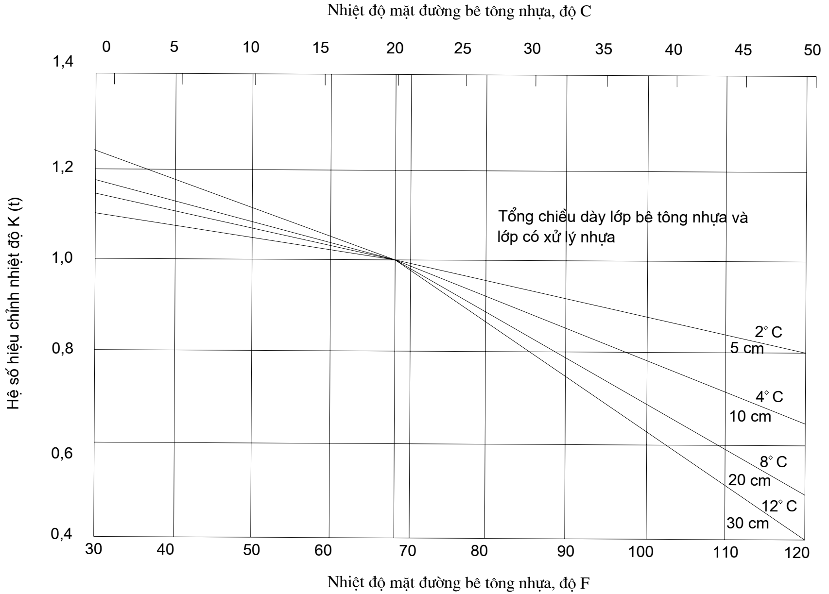
Hình 3. Hiệu chỉnh d của mặt đường bê tông nhựa về nhiệt độ tính toán khi lớp móng trên làm bằng vật liệu có gia cố xi măng
