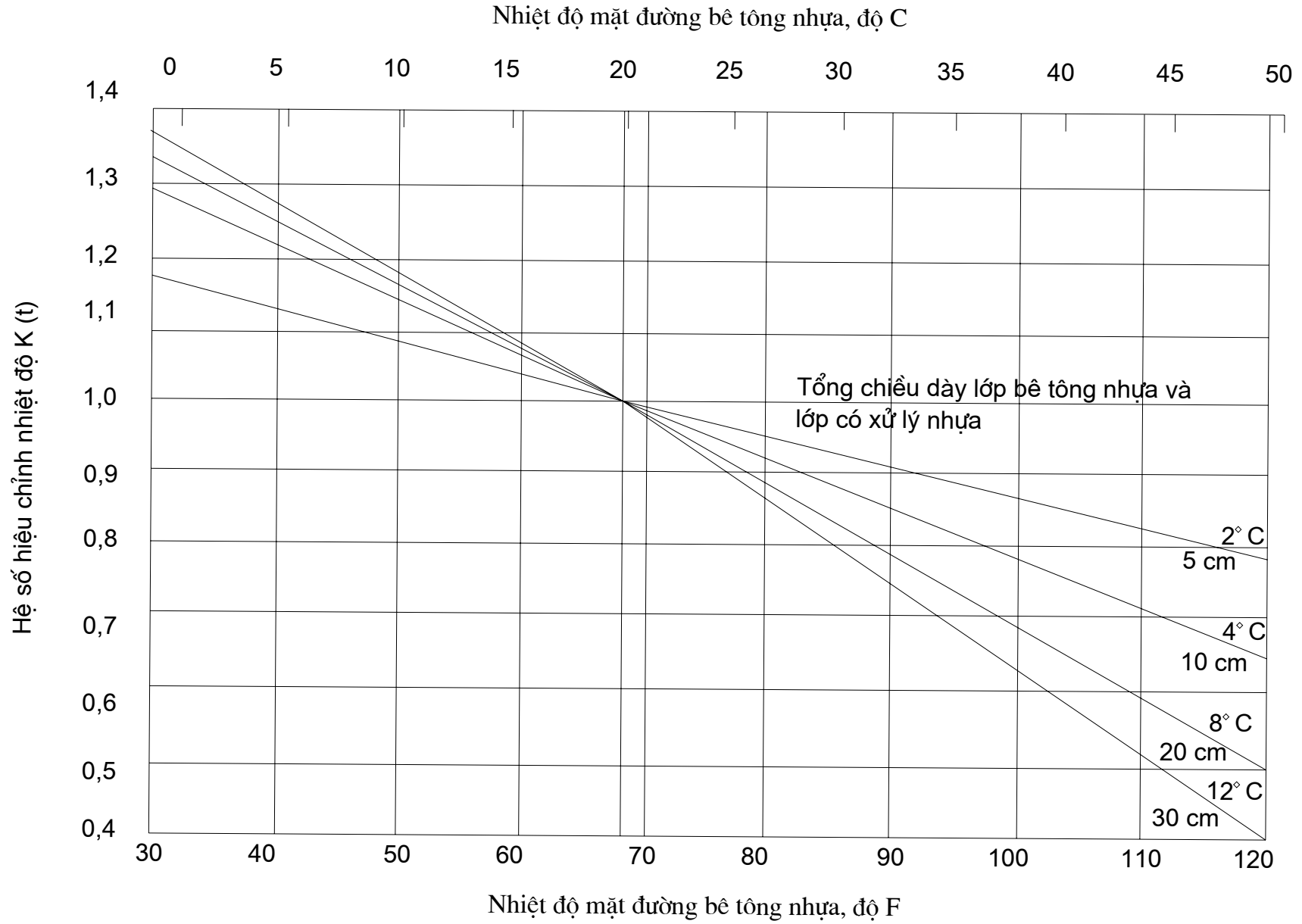
Hình 2. Hiệu chỉnh d. của mặt đường bê tông nhựa về nhiệt độ tính toán khi lớp móng trên là vật liệu hạt hoặc vật liệu có xử lý nhựa
