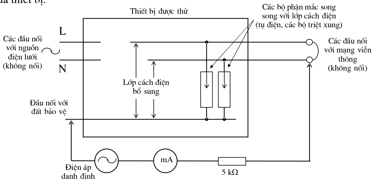
Hình 3 - Phép thử sự cách ly giữa mạng viễn thông và đất
