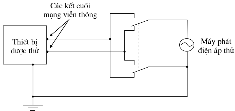
Hình 2 - Máy phát điện áp thử
