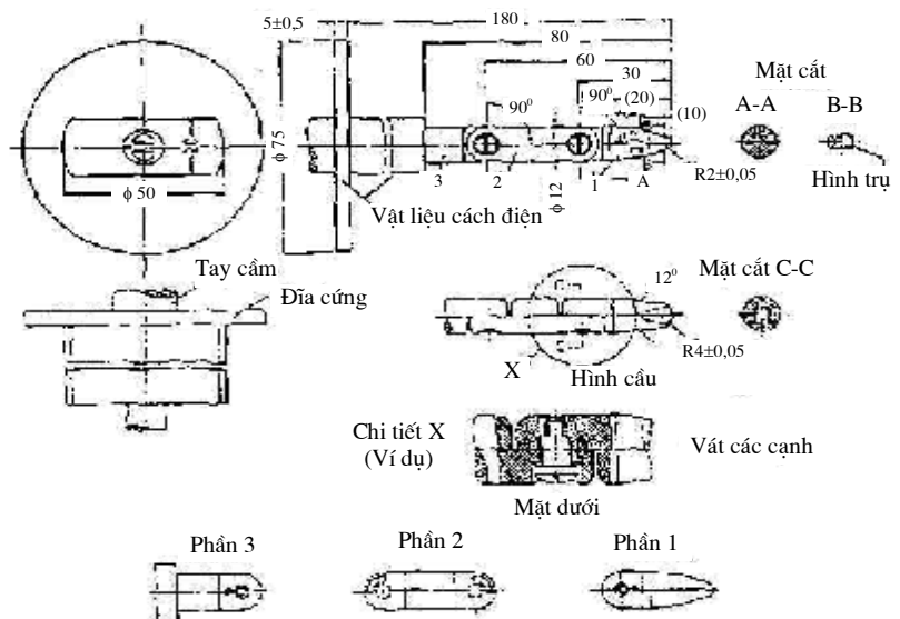
Hình E1 - Que thử (test probe)
