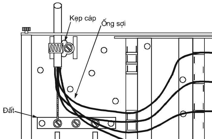
Hình C.9: Lắp đặt kẹp cáp
