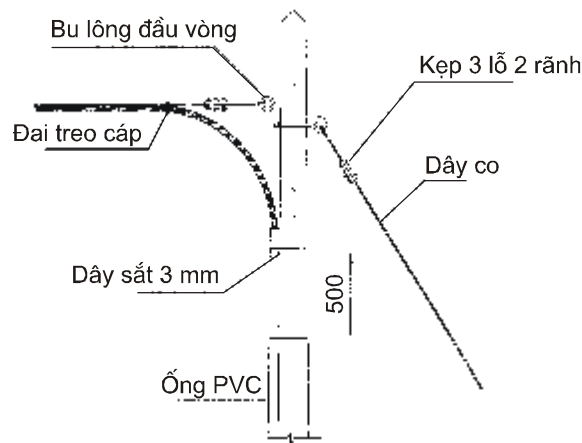
Hình C.1: Kết cuối dây treo cáp bằng bu lông đầu vòng
