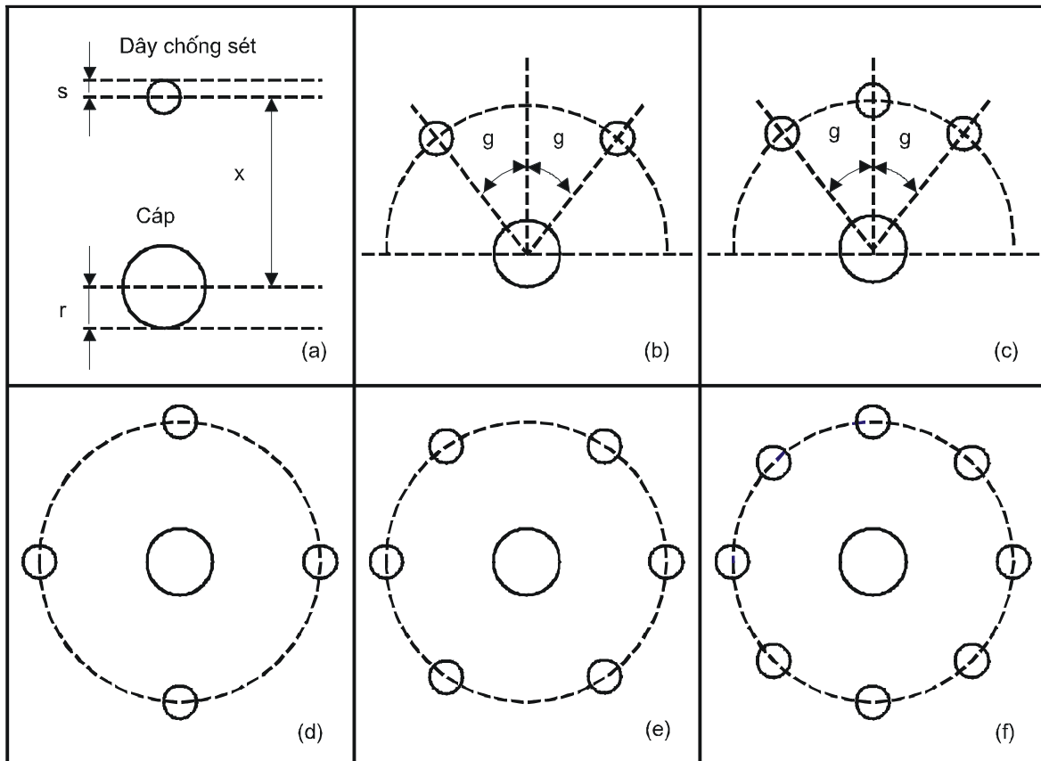
Hình B.1: Sắp xếp các dây chống sét ngâm bao bọc xung quanh cáp viễn thông
