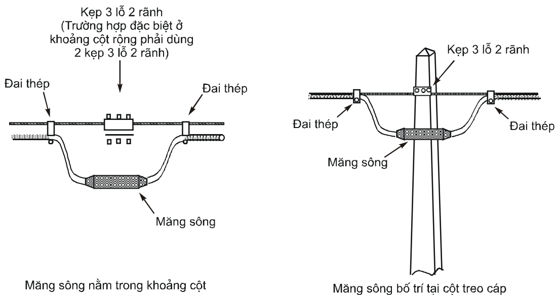
Hình C.4: Măng sông cáp treo
