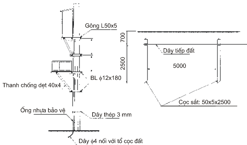
Hình C.3: Tiếp đất tủ cáp
