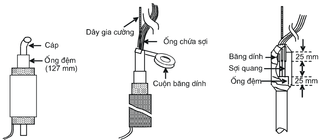
Hình C.8: Chuẩn bị đầu cáp
