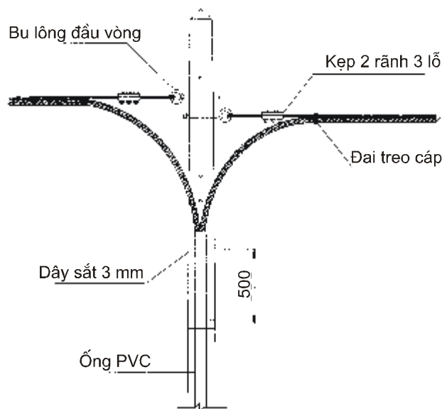
Hình C.2: Kết cuối dây treo cáp ở nơi cáp vào và ra tủ cáp
