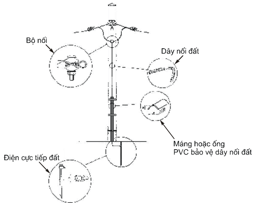
Hình C.10: Hệ thống nối đất dây thép bền treo cáp
