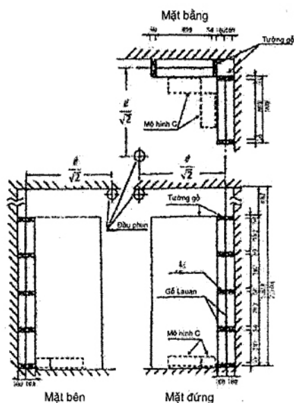
Hình 3 – Bố trí thử nghiệm 1, loại II
