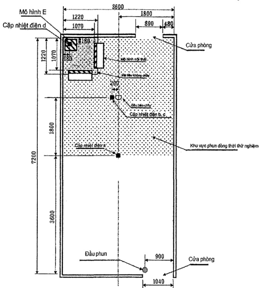
Hình 6 – Bố trí thử nghiệm khả năng ngăn cháy lan
