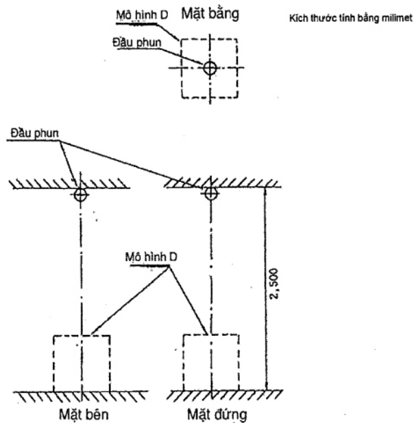
Hình 5 – Bố trí thử nghiệm 2, loại 2
