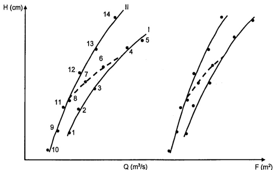
Hình 6 - Đường quan hệ Q = f(H) và đường chuyển tiếp khi bị ảnh hưởng phai
