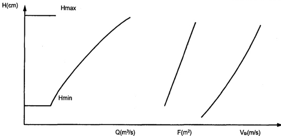
Hình 1 - Đường quan hệ Q = f(H) , F = f(H) , V_b = f(H)
