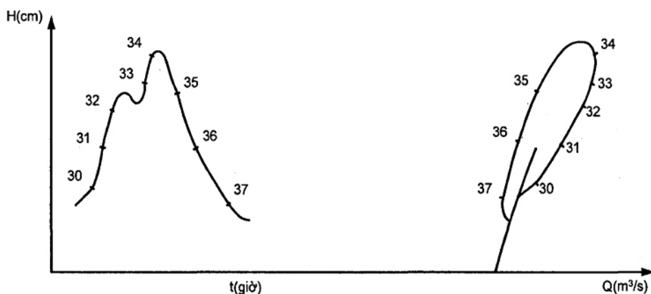
Hình 4 - Đường quan hệ H = f(t) (giờ) và Q = f(H) thời gian ảnh hưởng lũ
