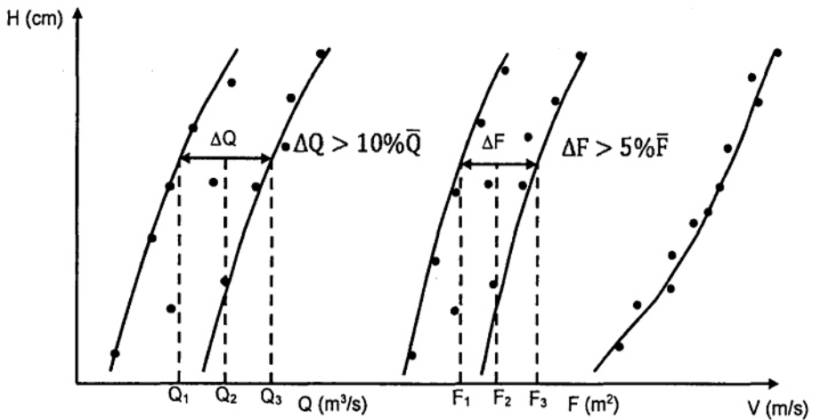
Hình 5 - Đường quan hệ Q = f(H) , F = f(H) , V_b = f(H) thời gian ảnh hưởng bởi xói
