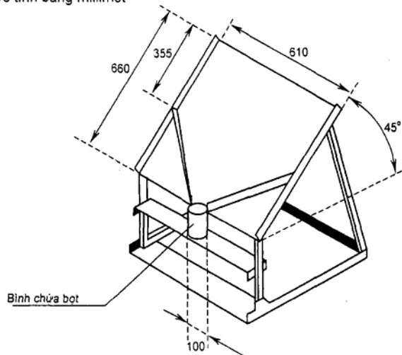
Hình 2 - Sơ đồ bộ phận thu bọt
