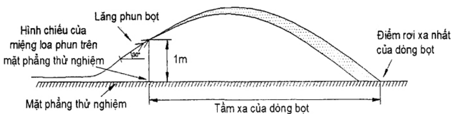
Hình 1 - Sơ đồ thử nghiệm tầm xa của dòng bọt
