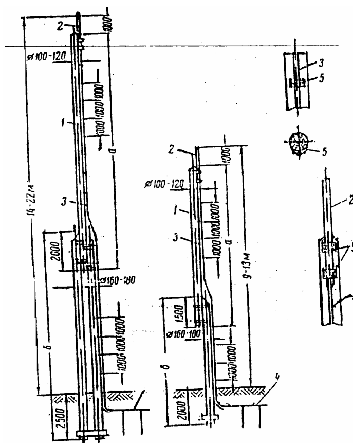
Hình 1.10 - Thu sét kiểu cột đặt trên cột đỡ bằng gỗ
