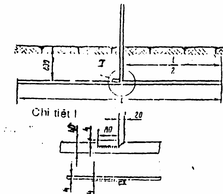
Hình I.15 - Tiếp đất kiểu dẹt hình tia chữ T
