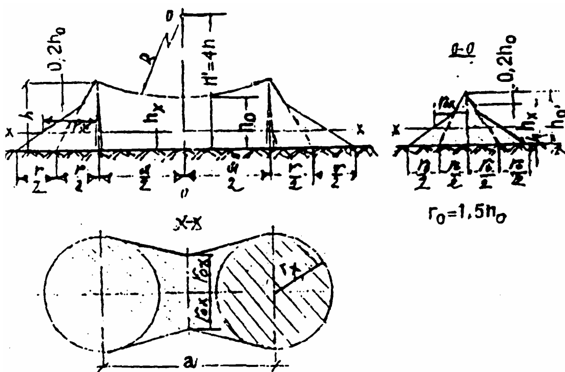
Hình 1.3 - Vùng bảo vệ của thu sét kép kiểu cột
