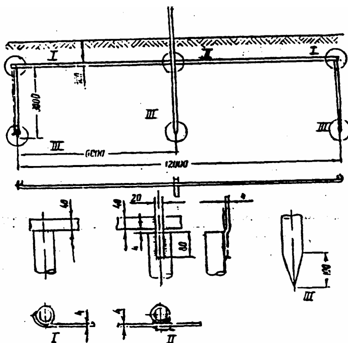
Hình 1.13 - Vật tiếp đất gồm 3 ống
