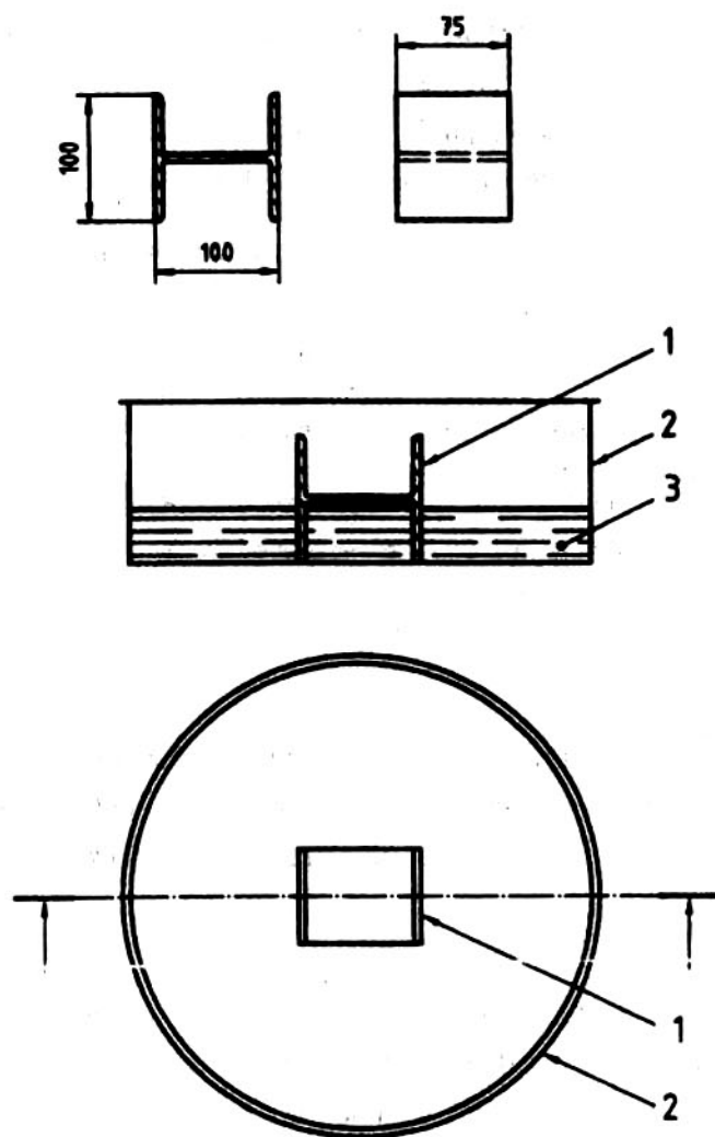
Hình 3 – Hình dạng đám cháy lan magie có vật cản
