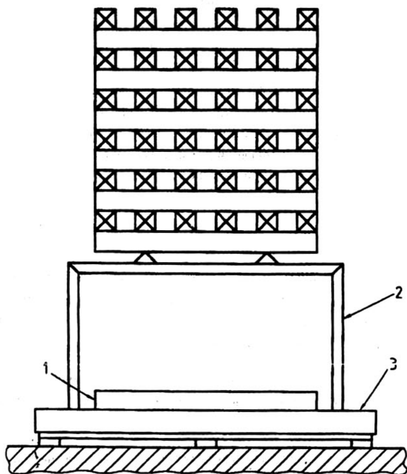
1 - Khay mỡ cháy; 2 - Khung đỡ; 3 - Bàn cân
