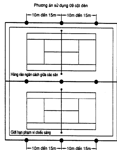
Hình 23 : Bố trí cột đèn chiếu sáng sân quần vợt có hàng rào ngăn cách
