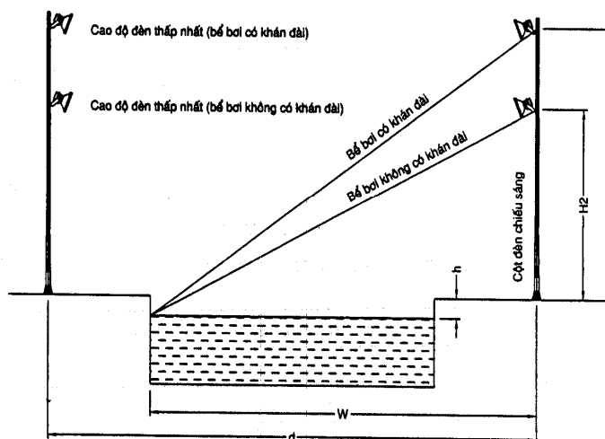
Hình 9 : Cao độ đặt đèn chiếu sáng bể bơi ngoài trời
