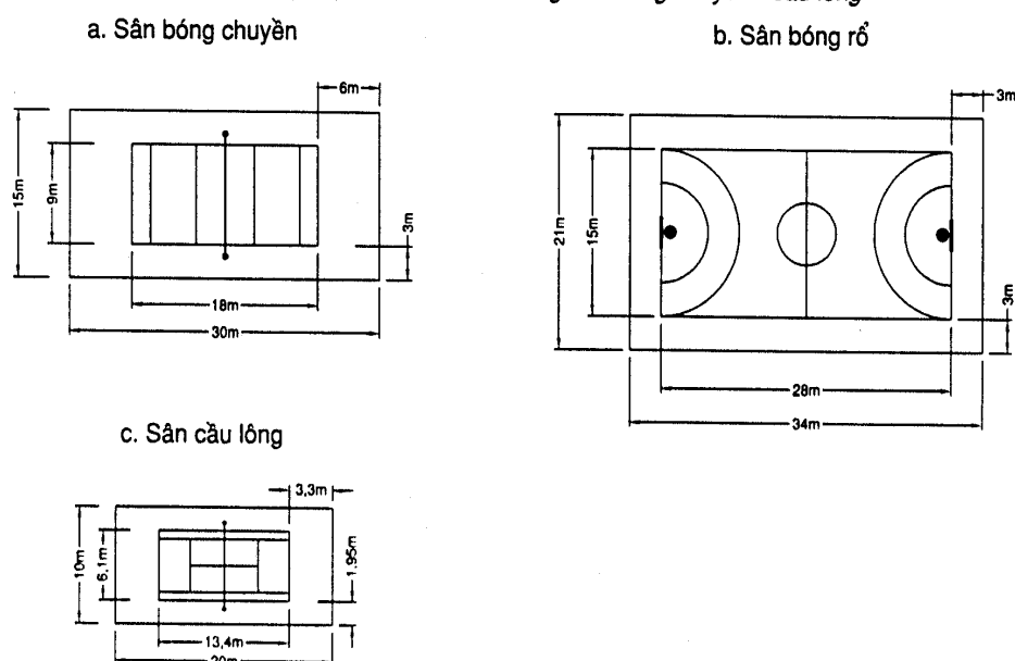
Hình 7 : Diện tích đo đạc và tính toán chiếu sáng sân bóng chuyên - cầu lông
