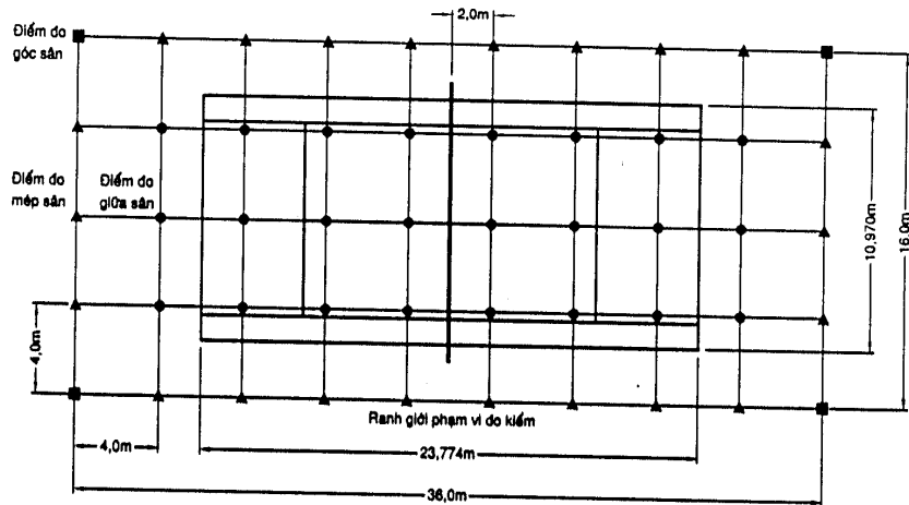
Hình 29 : Lưới đo kiểm chiếu sáng sân quần vợt
