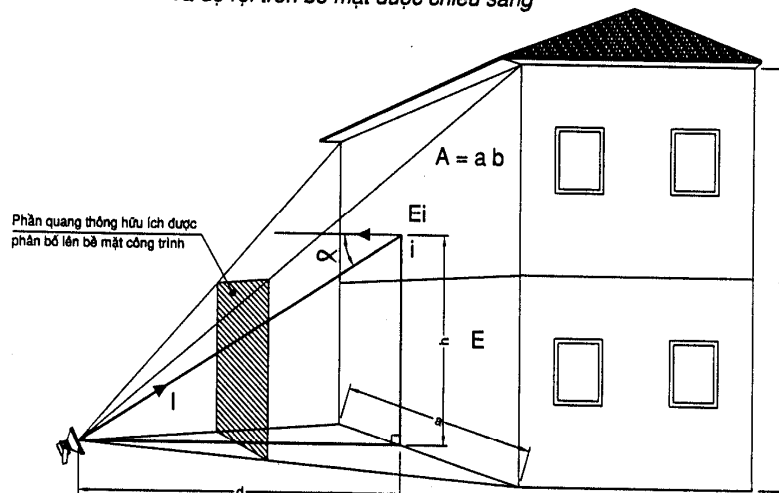
Hình 19 : Mối quan hệ giữa cường độ ánh sáng, khoảng cách chiếu sáng và độ rọi trên bề mặt được chiếu sáng
