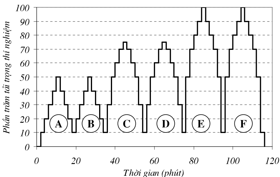
Hình B.1- Các cấp tải đối với thí nghiệm lập sáu chu kỳ
