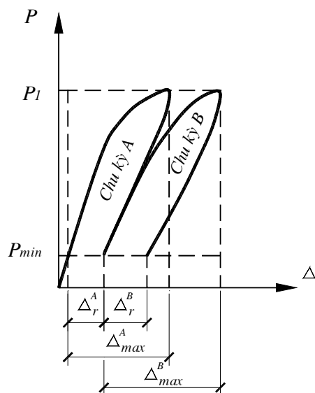
Hình B.2 - Xác định tính lặp của độ võng cho cặp chu kỳ A-B
