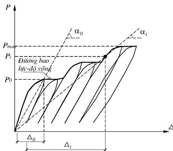
Hình B.3 - Xác định độ chênh tuyến tính tại điểm i
