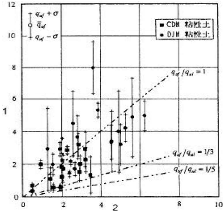
Hình B.3 - Quan hệ cường độ hiện trường và trong phòng (trên đất liên) (Sakai, 1996)
