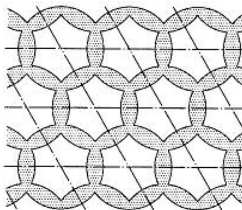
Hình A.6 - Thí dụ bố trí trụ trộn khô: 1 Dải; 2 Nhóm, 3 Lưới tam giác, 4 Lưới vuông
