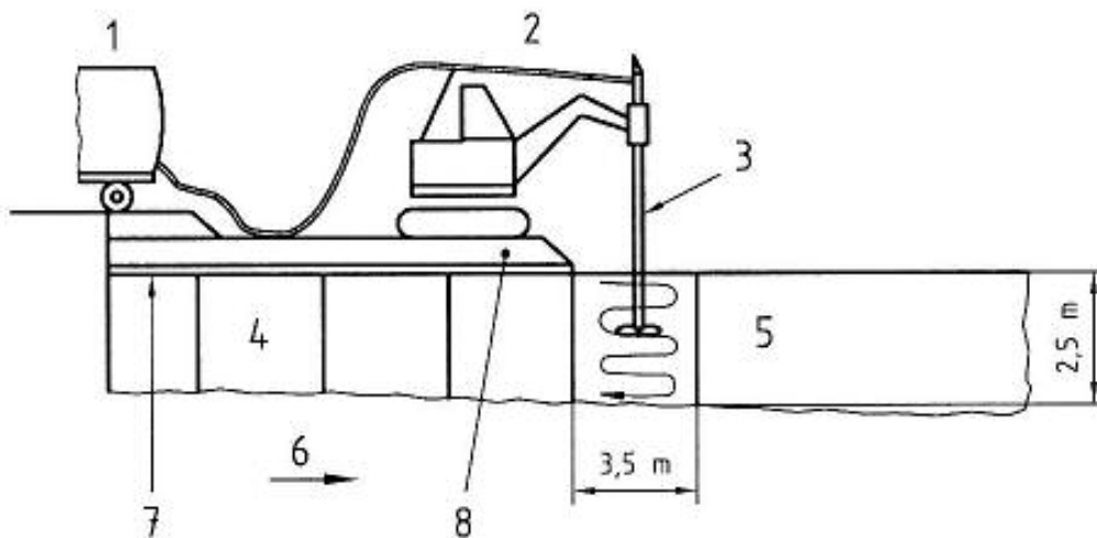
Hình A.11 - Ổn định khối kiểu A
