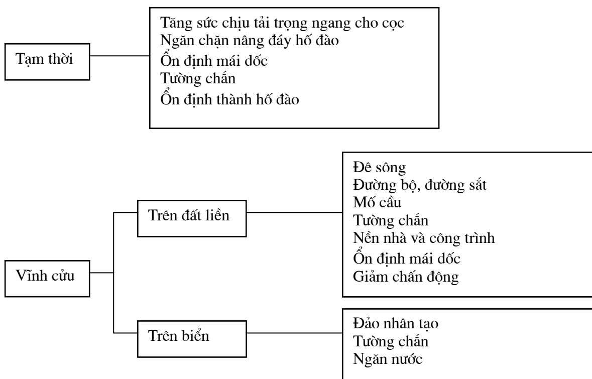
Hình A.2 - Ứng dụng trộn sâu
