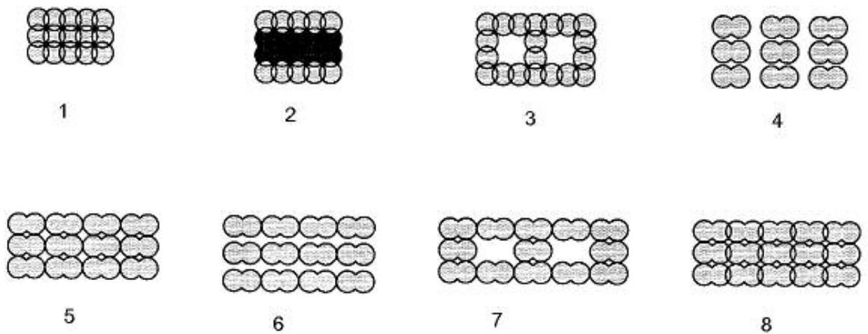
Hình A.9 - Thí dụ bố trí trụ trộn ướt trên biển: 1 Kiểu khối, 2 Kiểu tường, 3 Kiểu kẻ ô, 4 Kiểu cột, 5 Cột tiếp xúc, 6 Tường tiếp xúc, 7 Kẻ ô tiếp xúc, 8 Khối tiếp xúc
