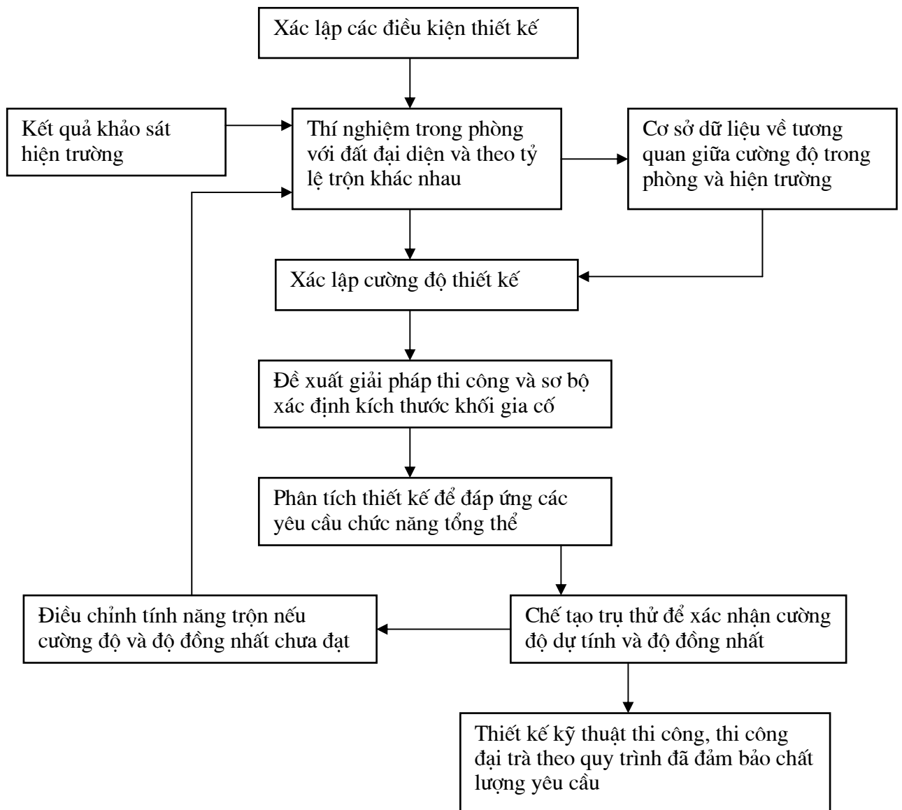
Hình B.1 - Quy trình thiết kế lập, gồm thí nghiệm trong phòng, thiết kế chức năng, thử hiện trường và thiết kế công nghệ
