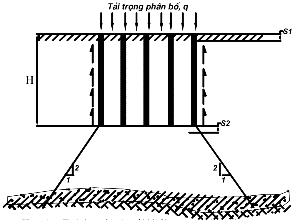
Hình C.1 Tính lún nền gia cố khi tải trọng tác dụng chưa vượt quá sức chịu tải cho phép của vật liệu trụ
