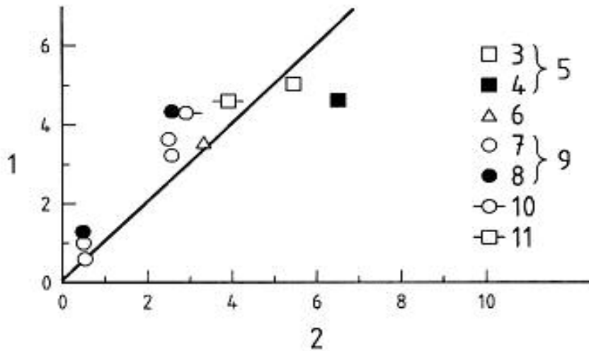
Hình B.3 - Quan hệ cường độ hiện trường và trong phòng (trên đất liên) (Sakai, 1996)
