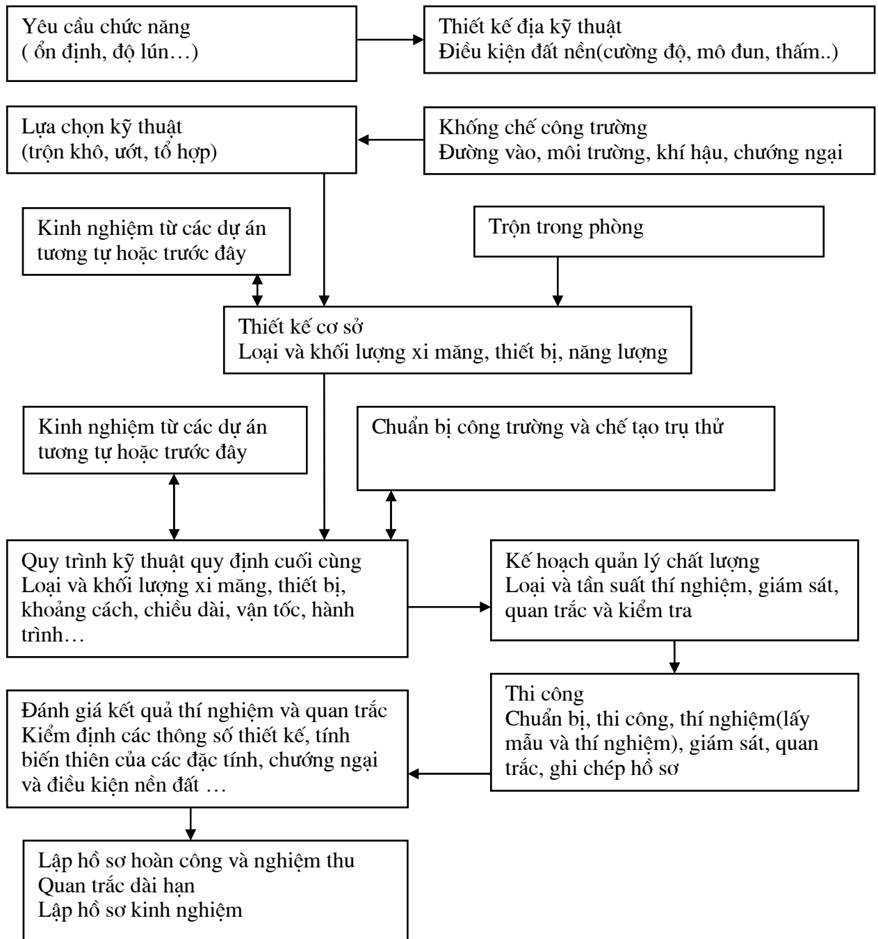
Hình A.3 - Nguyên tắc thực hiện dự án thi công trộn sâu
