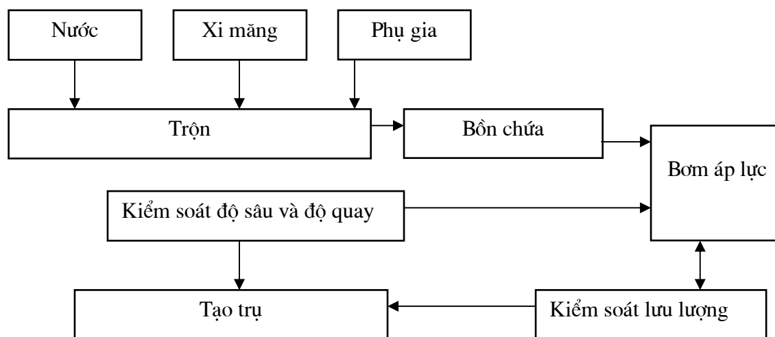
Hình A.5 - Sơ đồ thi công trộn ướt
