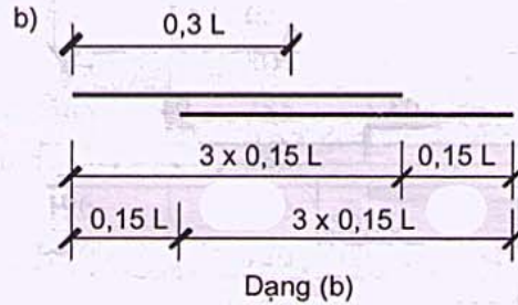
Hình E.4: Lưới thép bố trí thành 2 lớp để chịu mô men âm ở vùng gối của sàn
