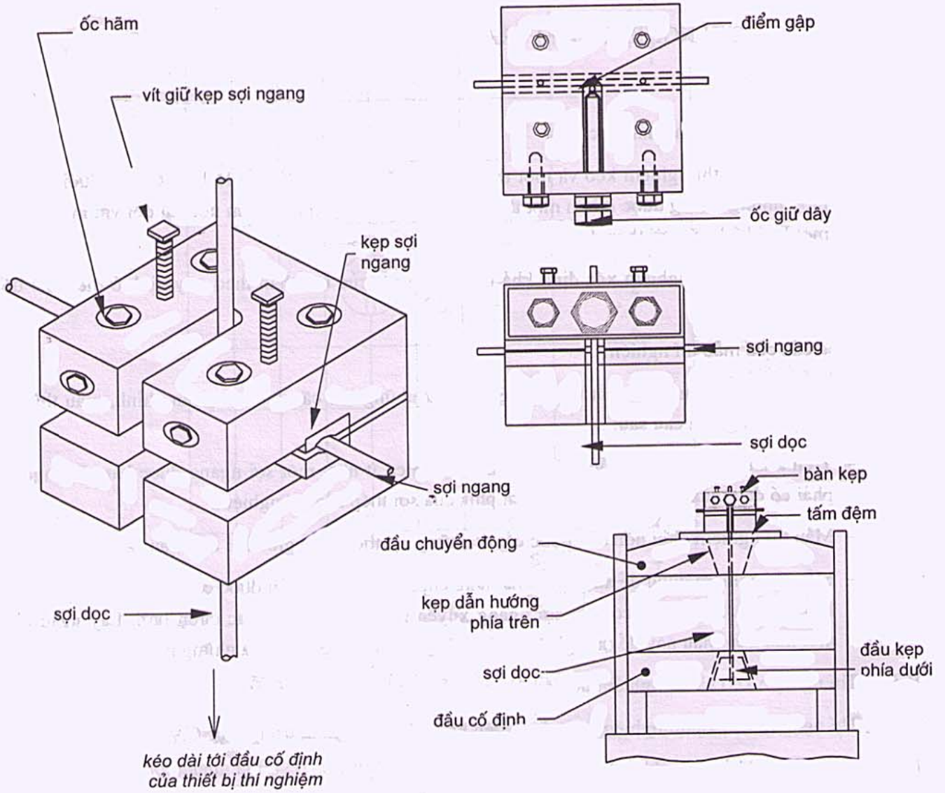
Hình B.1: Sơ đồ thí nghiệm cường độ chịu cắt của mối hàn.
