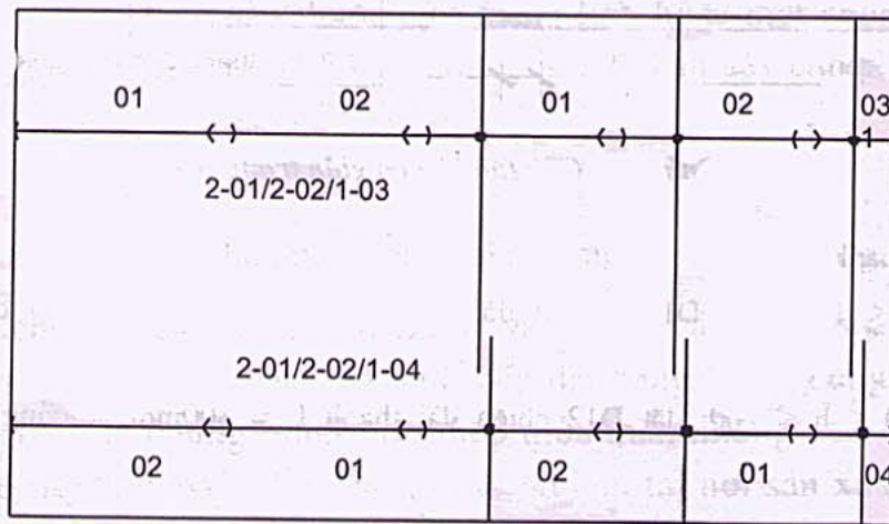
Hình D.2: Ví dụ thể hiện lưới thép hàn trên bản vữa
