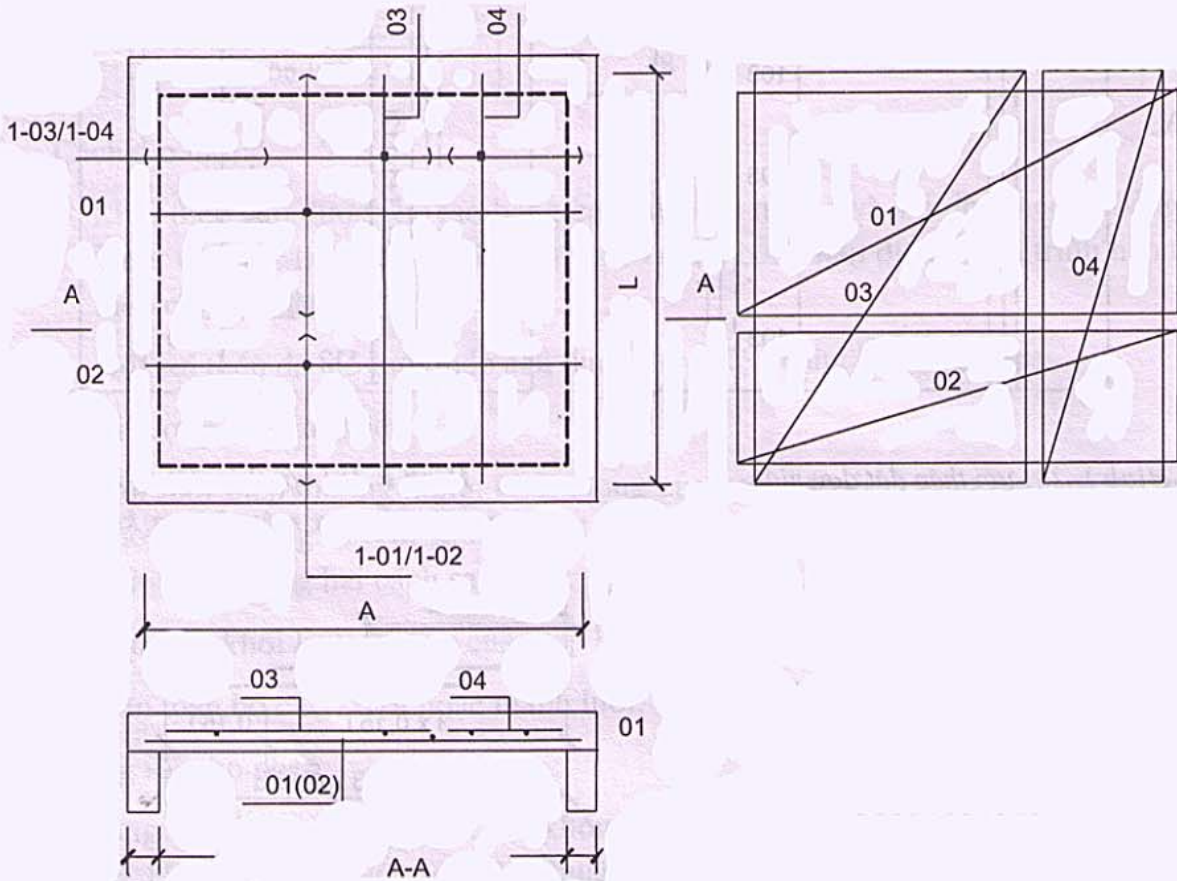
Hình E.6: Lưới thép trong sàn chịu lực 2 phương, gối đơn giản
