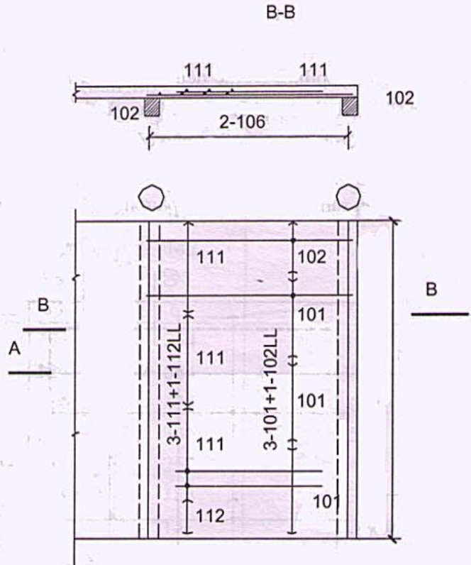
Hình E.3: Lưới thép đặt so le trong sàn chịu lực một phương, kê tự do
