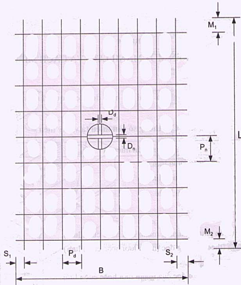
Hình A.1: Các ký hiệu trên một mảnh lưới
