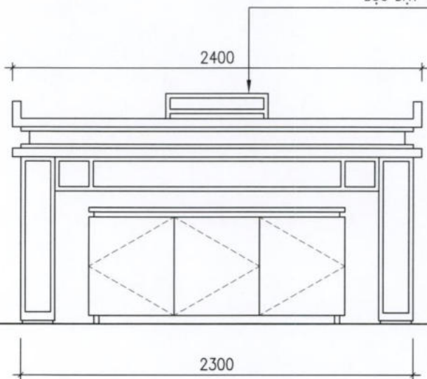
MẶT ĐỨNG CHÍNH
