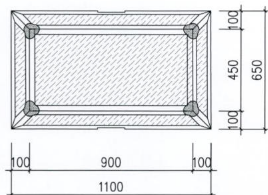
MẶT BẰNG LỒNG KÍNH
