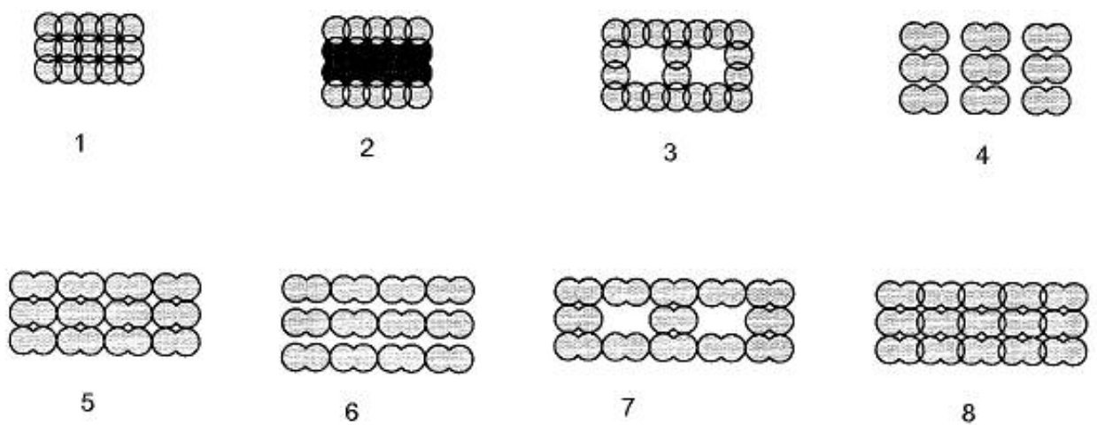
Hình A.9 - Thí dụ bố trí trộn ướt trên biển: 1 Kiểu khối, 2 Kiểu tường, 3 Kiểu kẻ ô, 4 Kiểu cột, 5 Cột tiếp xúc, 6 Tường tiếp xúc, 7 Kẻ ô tiếp xúc, 8 Khối tiếp xúc
