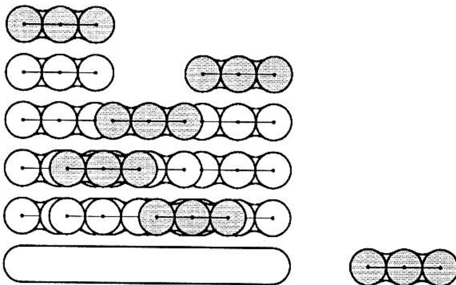
Hình A.10 - Thí dụ bố trí trộn ướt chồng nhau trộn ướt, thứ tự thi công
