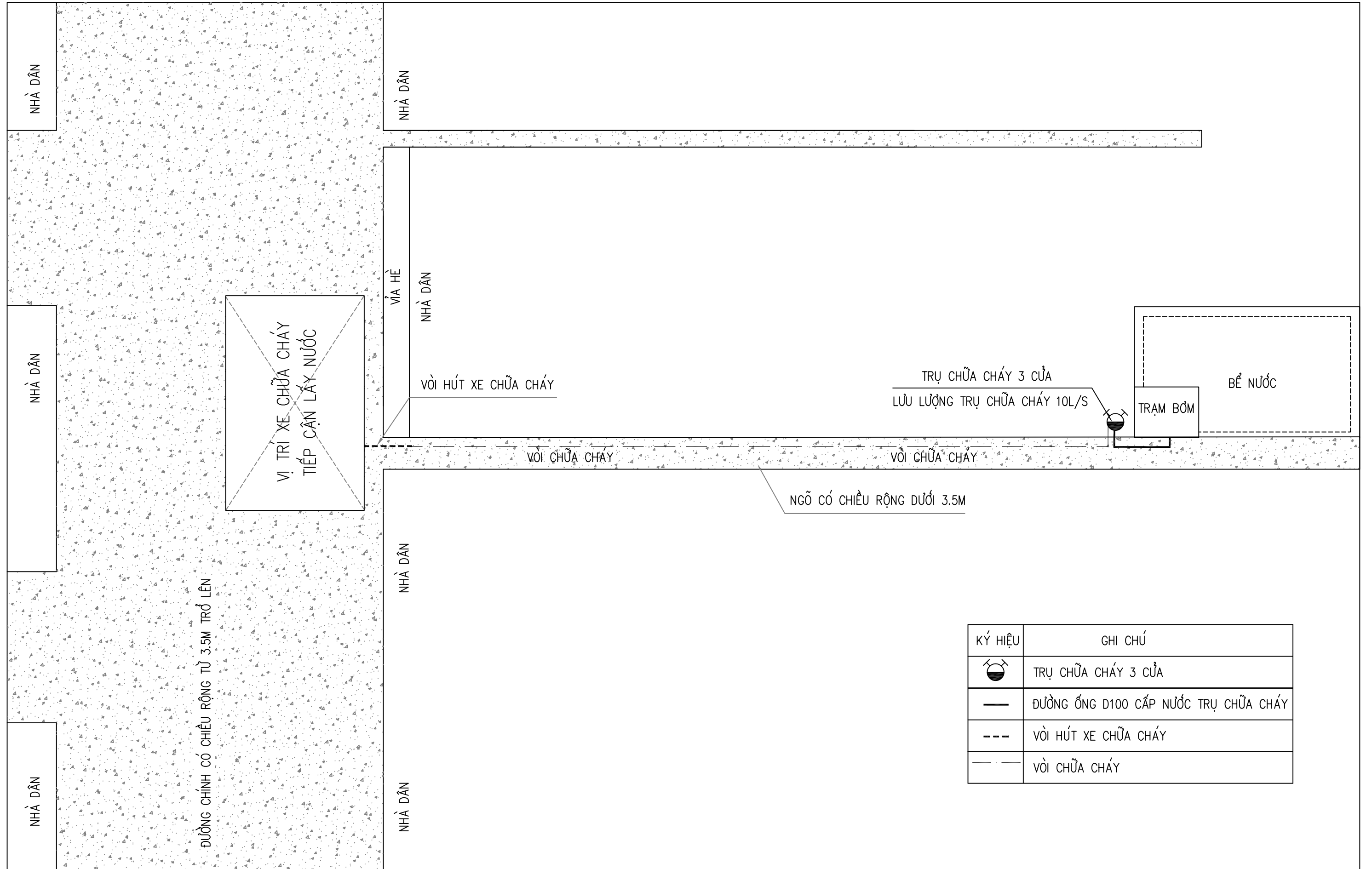
PHƯƠNG ÁN 2 TRƯỜNG HỢP 1 XE CHỮA CHÁY CÓ THỂ TIẾP CẬN LẤY NƯỚC TỪ TRỤ CHỮA CHÁY (HÌNH 2)
