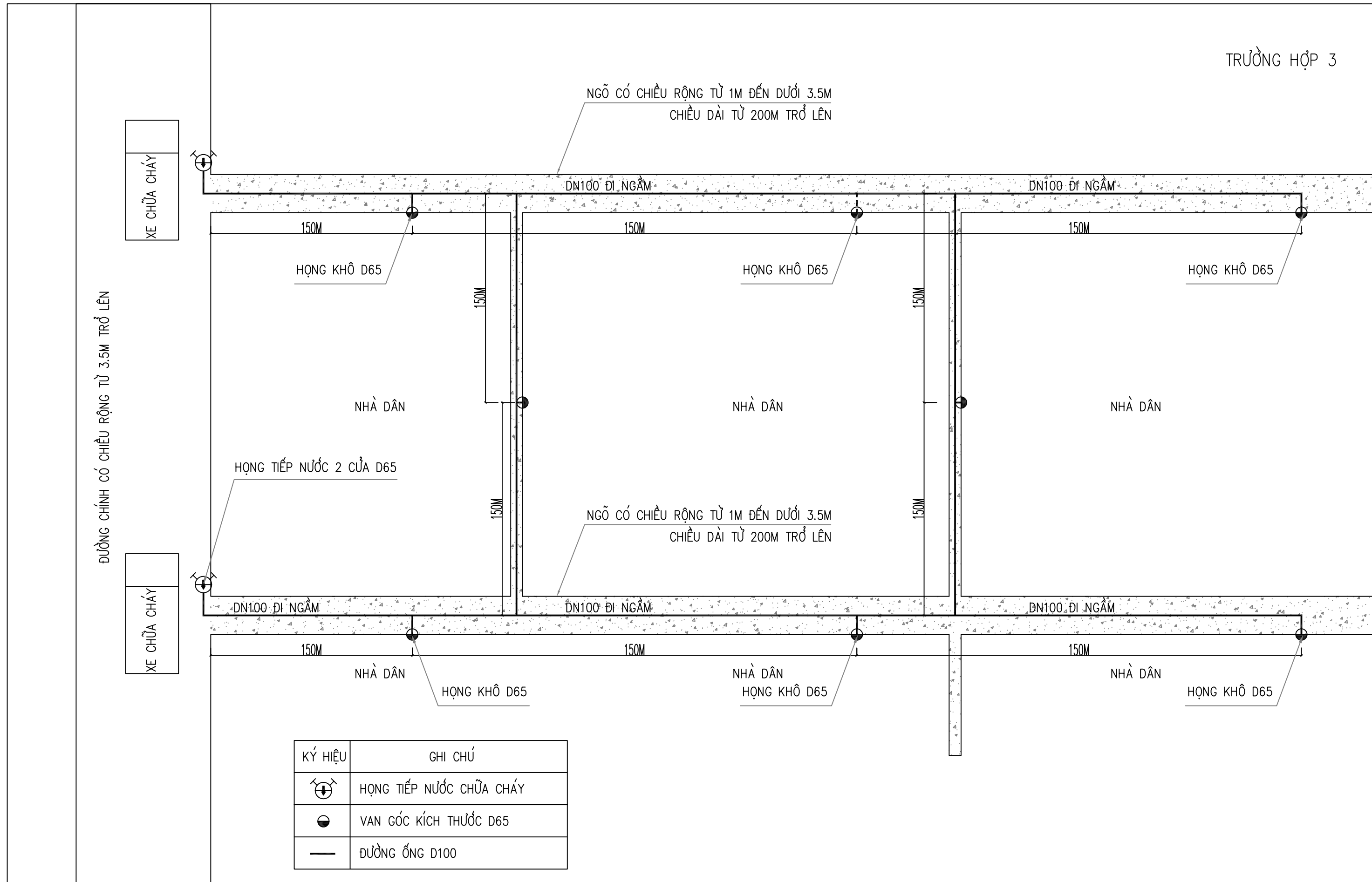
PHƯƠNG ÁN 2 TIẾP NƯỚC TỪ XE CHỮA CHÁY ĐỂ CẤP CHO ĐƯỜNG ỐNG HỌNG KHÔ LẤP ĐẶT TRONG NGÕ SÂU(HÌNH 3)
