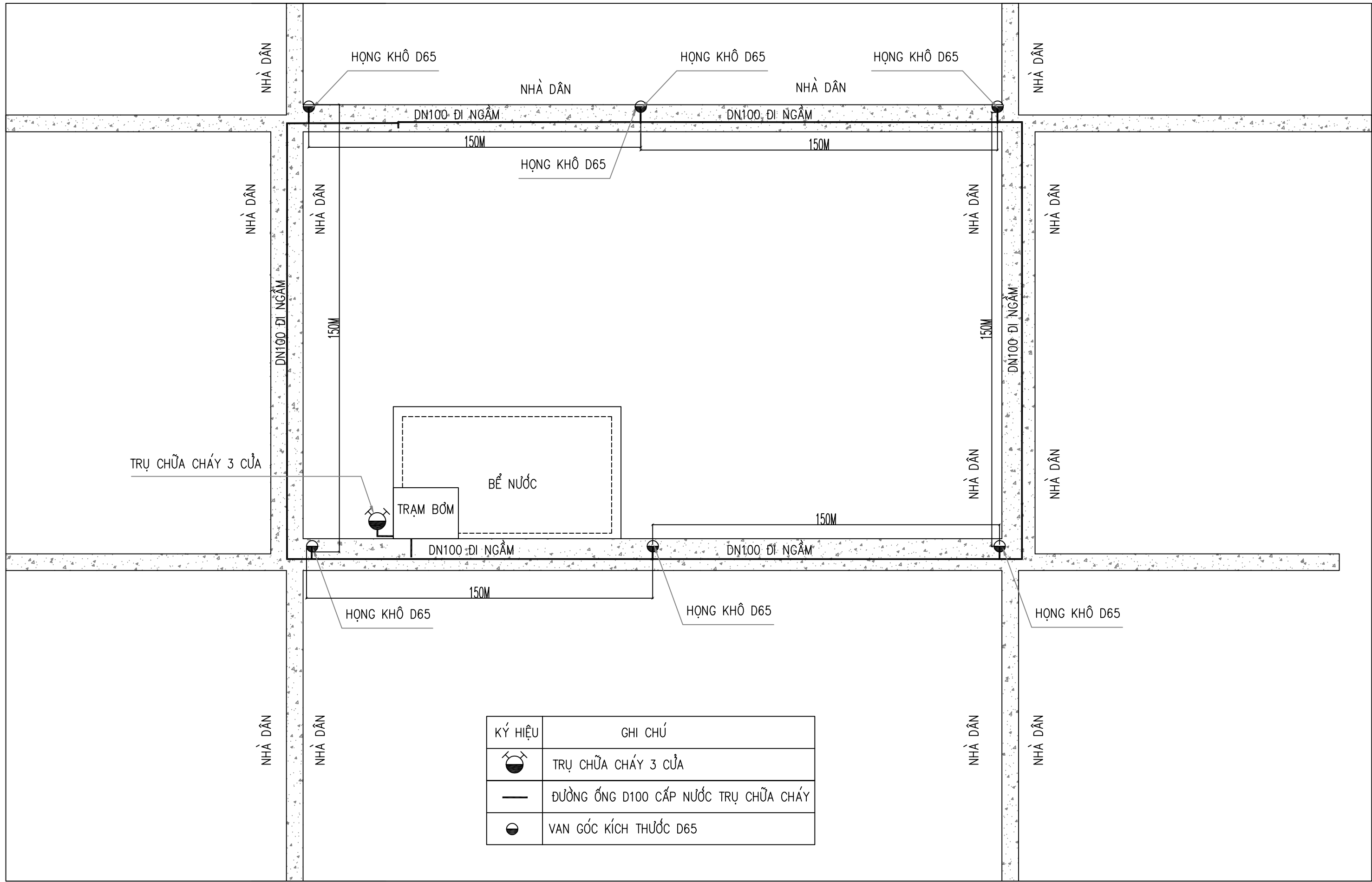
PHƯƠNG ÁN 1 TRẠM BƠM ĐẤU NỐI TRỰC TIẾP VÀO HỆ THỐNG ĐƯỜNG ỐNG CẤP NƯỚC NGÕ SÂU
