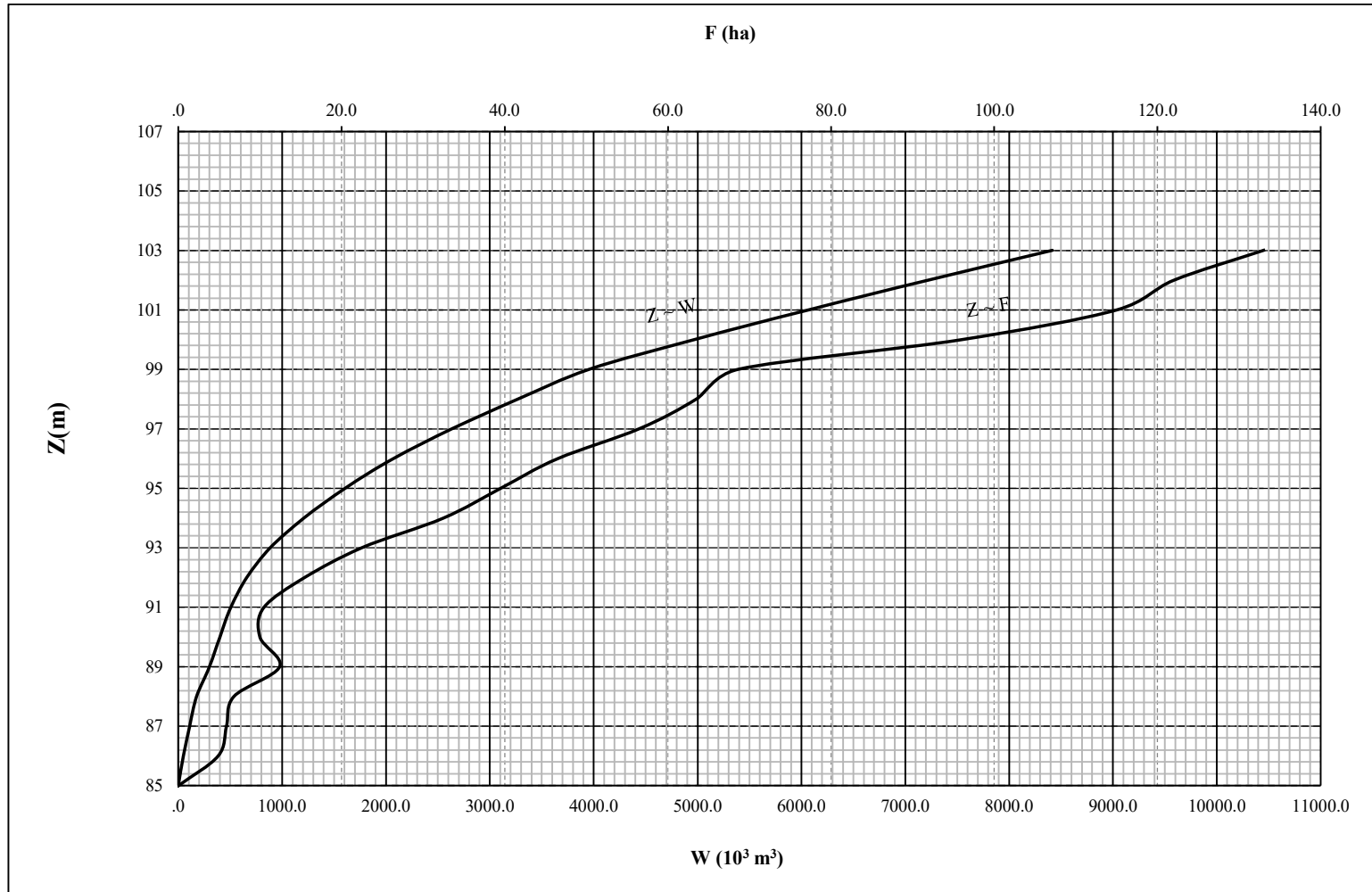
Hình II-3: Biểu đồ quan hệ mực nước, dung tích, diện tích mặt hồ
