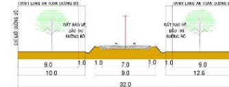
IV-IV ĐƯỜNG CẤP IV
