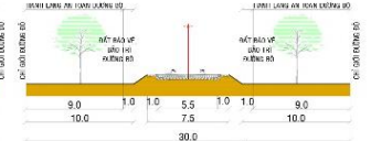
V-V ĐƯỜNG CẤP V
