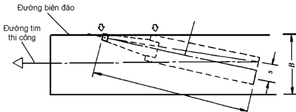
Hình 1. Chiều rộng nạo vét nhỏ nhất khi độ sâu nước hai bên luồng đào nhỏ hơn mớn nước
