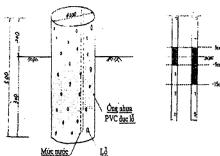
Hình A.2 - Lắp đặt ống quan sát mực nước trong ô ruộng
