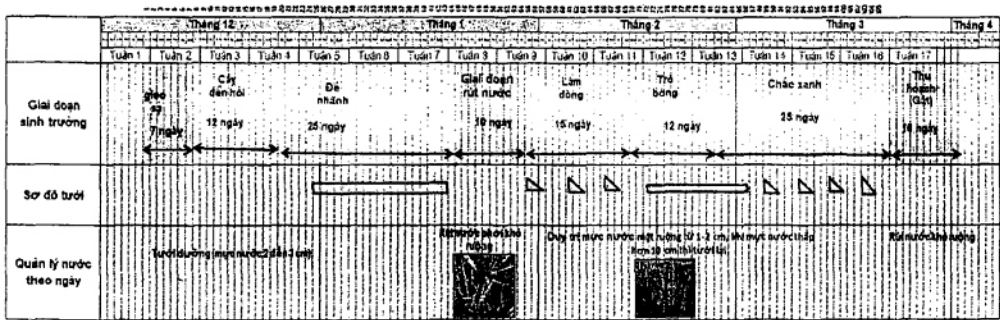
Hình 3 – Sơ đồ quy trình tưới tiết kiệm nước cho lúa, giảm phát thải khí mê tan vụ Đông Xuân vùng đồng bằng sông Cửa Long
