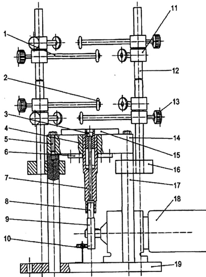
a) Sơ đồ chung
