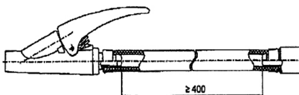
Hình 8 - Chiều dài nhỏ nhất của ống mềm
