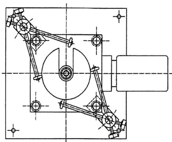
b) Hình chiếu nhìn từ trên xuống
