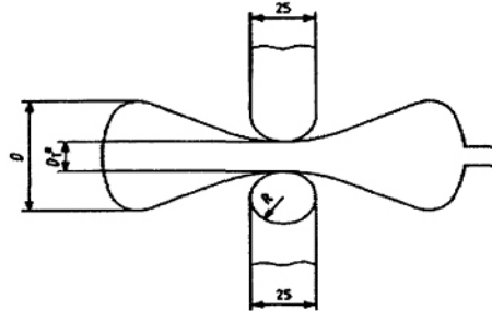
Hình 7 - Thử nén ép
