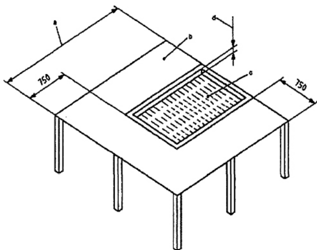
a) Các loại đấm cháy 15F, 25F và 75F
