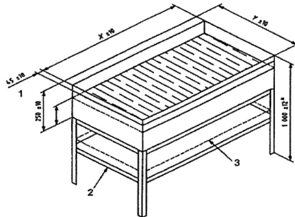
Hình 4- Các kích thước chung đối với thiết bị thử đám cháy loại F - Thiết bị thử kiểu A chỉ dùng cho loại đám cháy 5F
