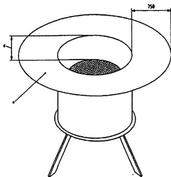
b) Loại đấm cháy 5F
