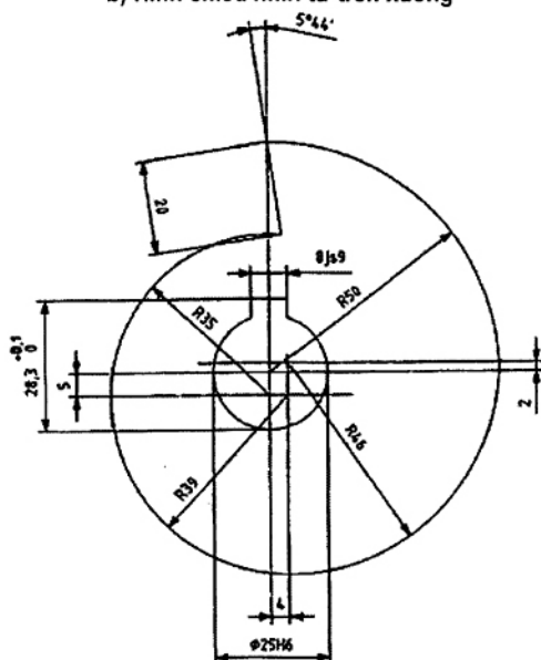
b) Hình chiếu nhìn từ trên xuống
