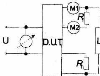
Hình 2b – Mạch điện thử nghiệm trở kháng balát
