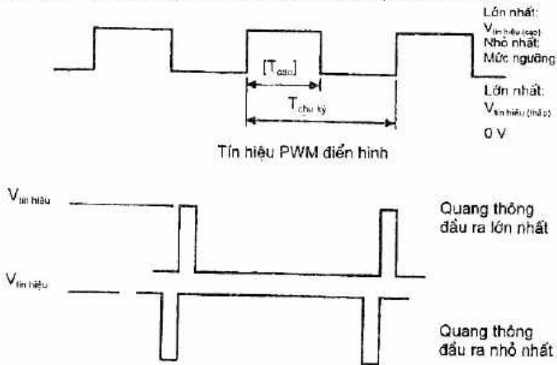
Tín hiệu PWM đối với quang thông đầu ra lớn nhất và nhỏ nhất
