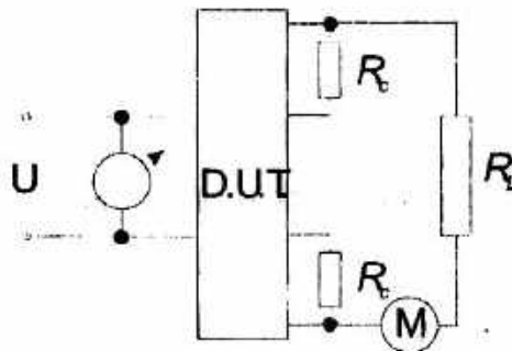
Hình 2a – Mạch điện thử nghiệm điện áp mạch hở
