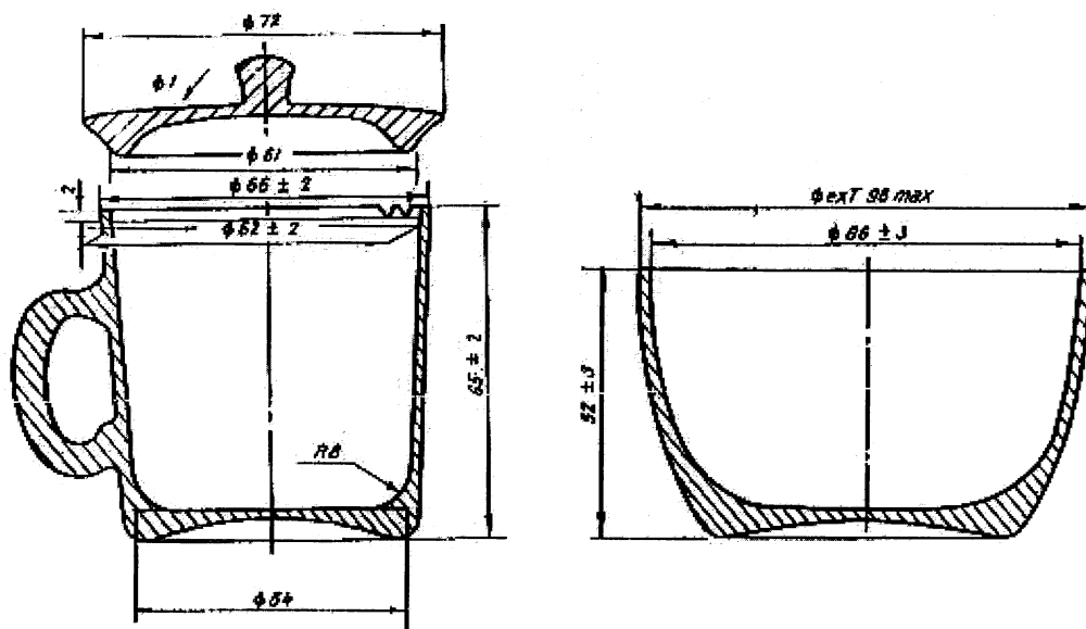
Hình 1 – Bộ ấm chén thử chè
