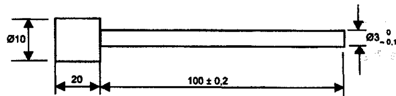
Hình 101 – Que thử đối với khóa liên động kín
