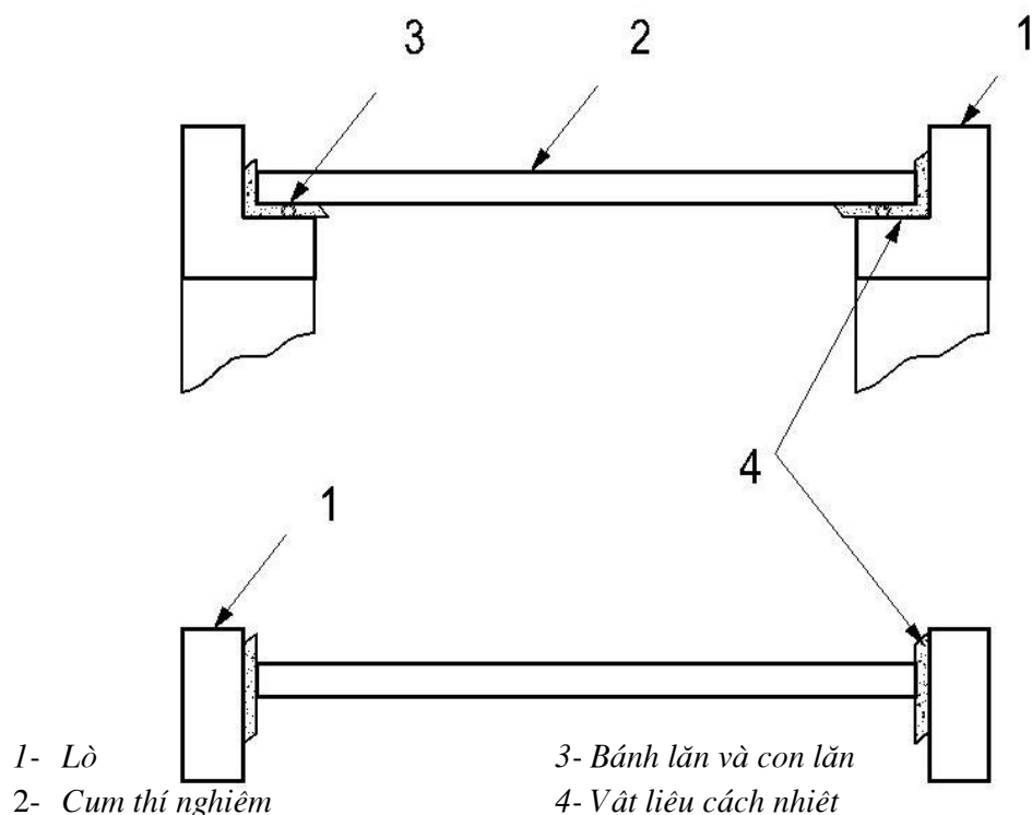
Hình 1 - Ví dụ về một mẫu thử tựa đơn giản đặt trong lò.
