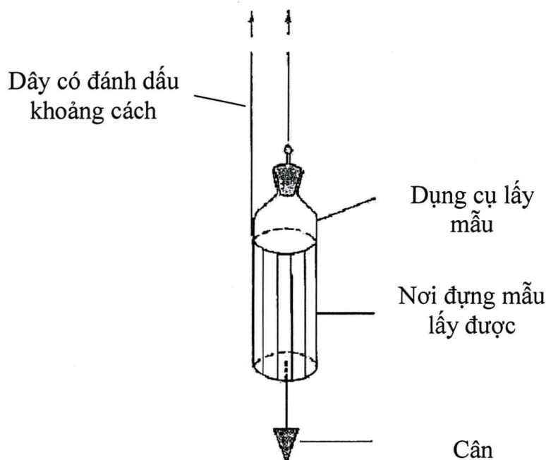
Hình 4. Dụng cụ lấy mẫu có thể cân được (weigntea container)
