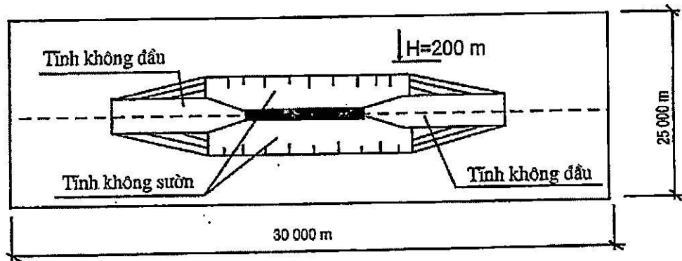
Hình 7-PLI: Vùng phụ cận đường sân bay
