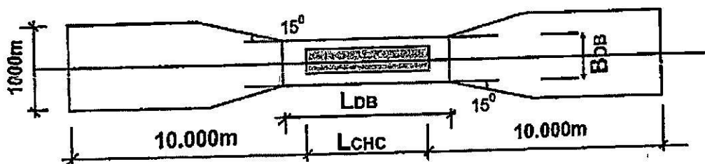
Hình 8b-PLI: Mặt bằng dải tính không đầu đường sân bay
