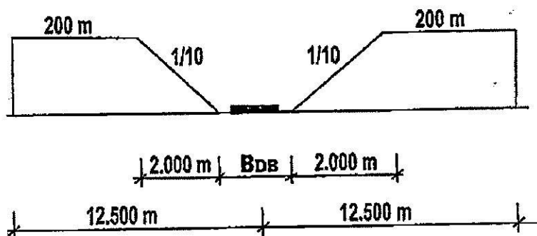
Hình 9-PLI: Kích thước dải tính không sùan đường sân bay
