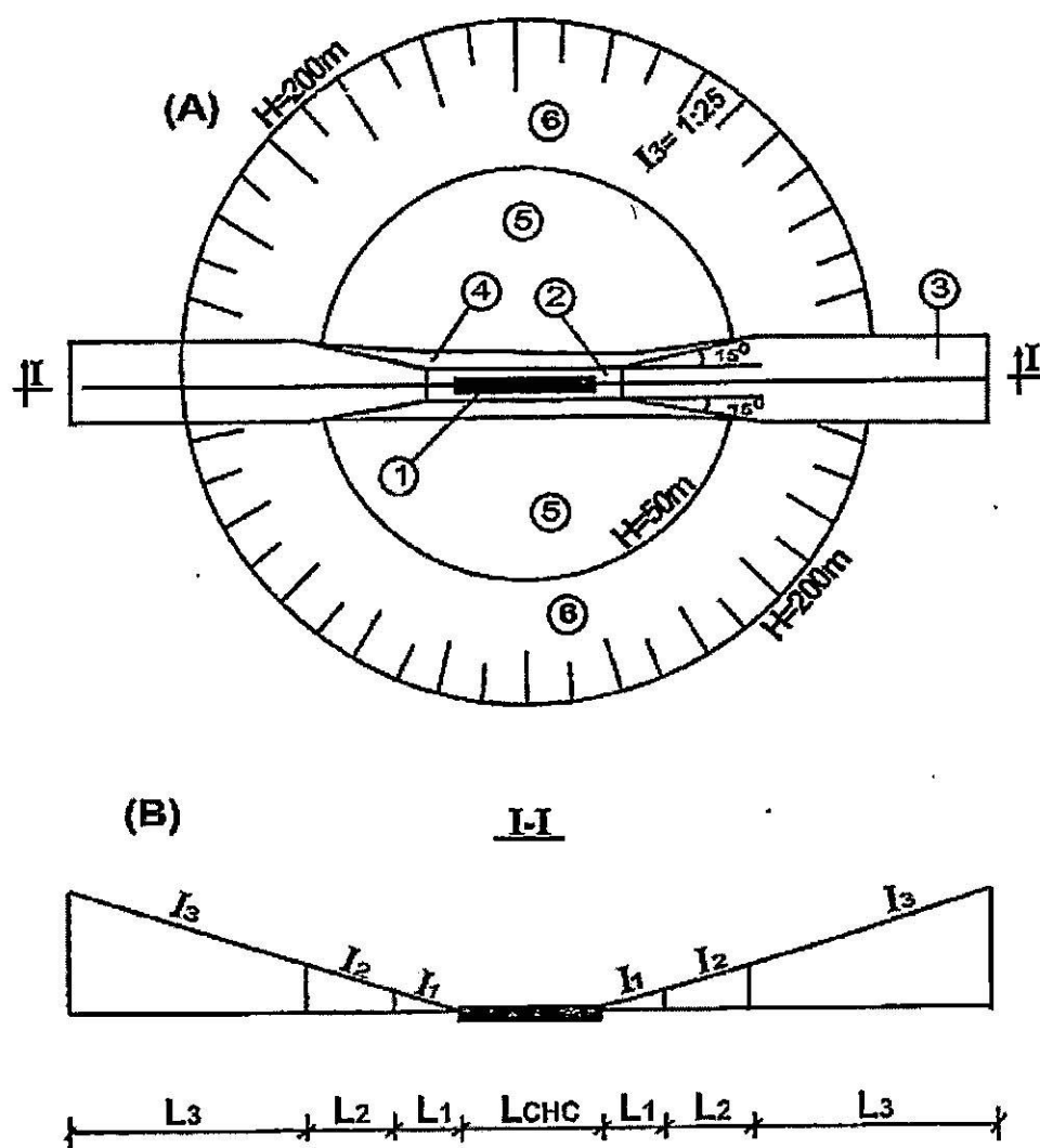
Hình 3a-PLI: Mặt bằng dài phụ cận đầu sân bay quân sự trong trường hợp có vòng lượn kín hẹp ở độ cao rất thấp
