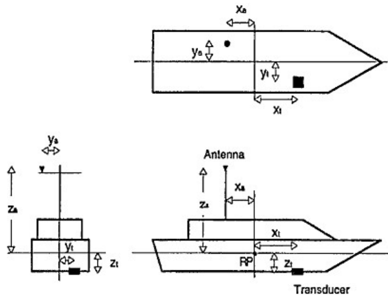
Ví dụ về đo các giá trị bù trừ (offset) của các thiết bị
