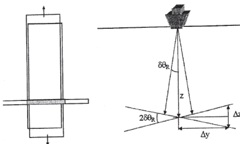
Hình 7: Xác định độ lệch nghiêng ngang
