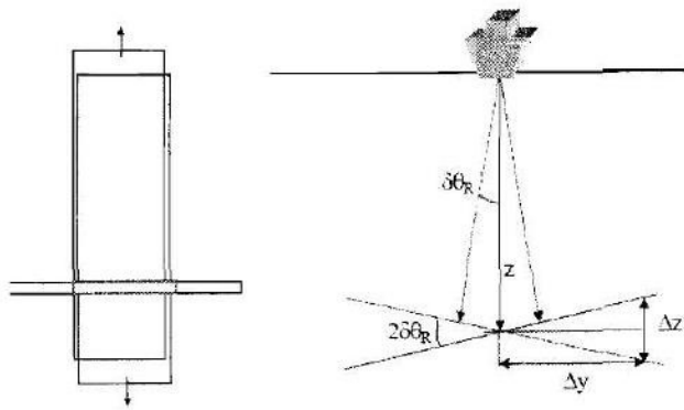
Hình 5: Xác định độ lệch nghiêng ngang
